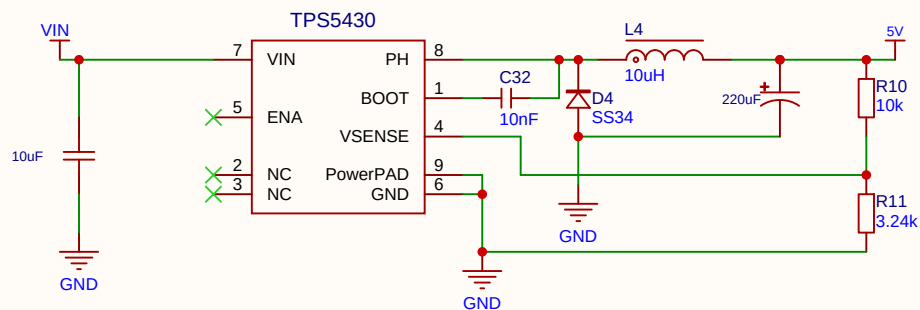
电源降压
