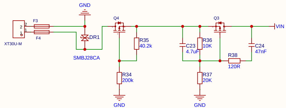
防反接软启动
