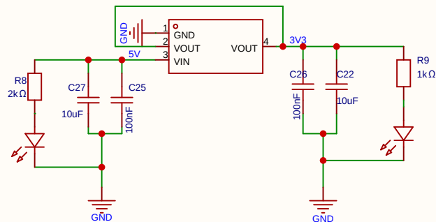
AMS1117-3.3_C6186
