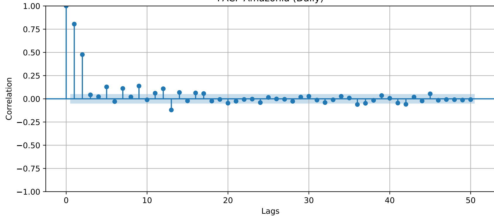
PACF Amazônia (Daily)
