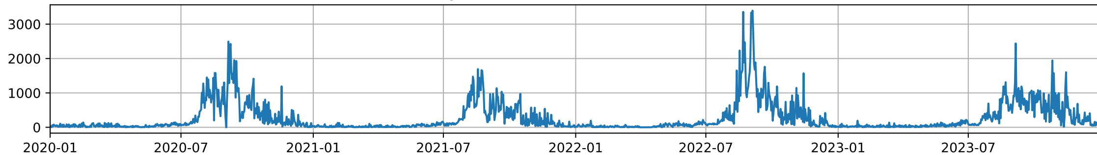
Trend (Amazônia biome)
