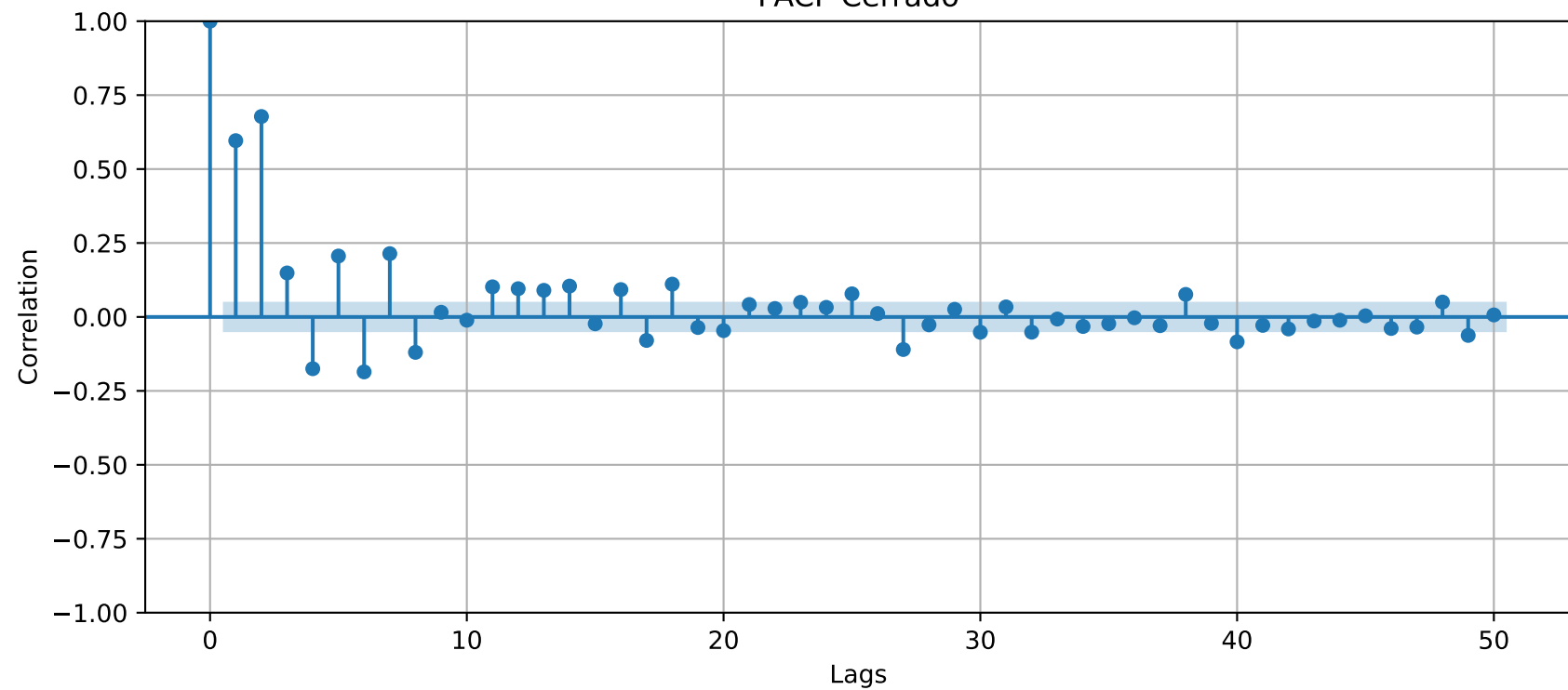
PACF Cerrado
