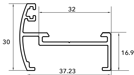
7201 MARCO
