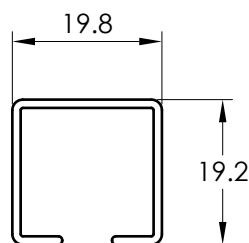
5322 RIEL PLUMILLA
