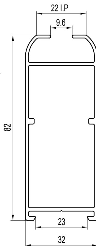
7202 BASTIDOR
