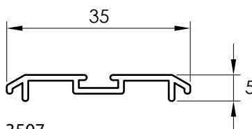
3507 TAPA PORTAFELPA
