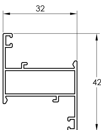
3202 HOJA
