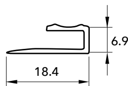
5361 TERMINACION
