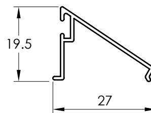
4229 JUNQUILLO MONOLITICO
