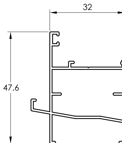
3205 MARCO CAMARA DE AGUA
