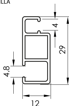
4220 ESCUADRA ANUDAL
