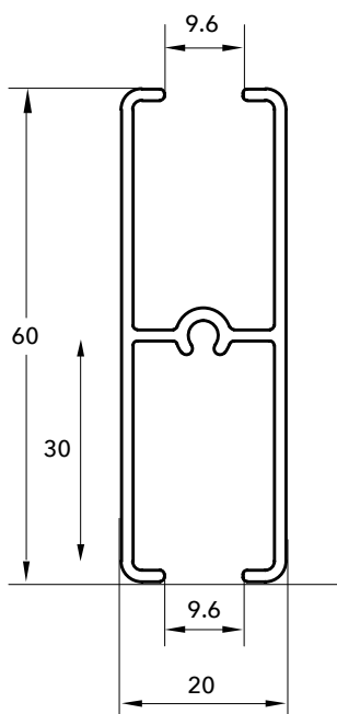
7206 PALILLO
