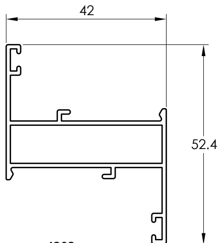
4202 HOJA
