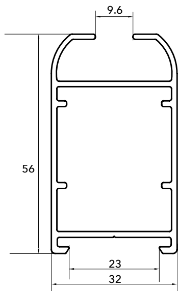
7202 BASTIDOR
