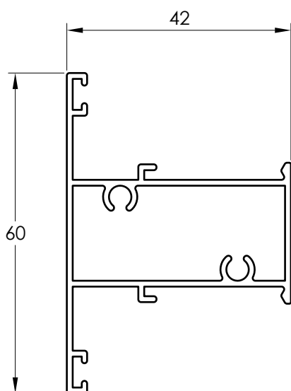
4204 PALILLO
