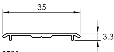
3506 TAPALISA
