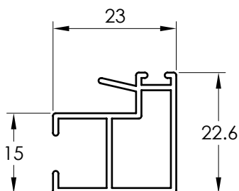
1508 TRASLAPO
