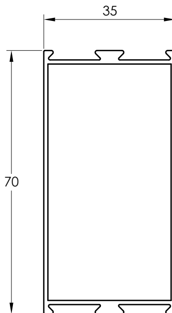
3501 BASTIDOR
