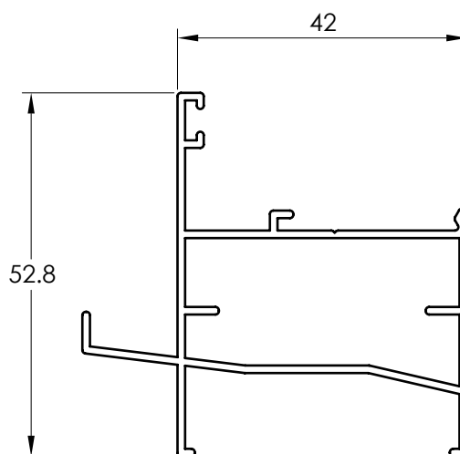
4231 MARCO CÁMARA DE AGUA
