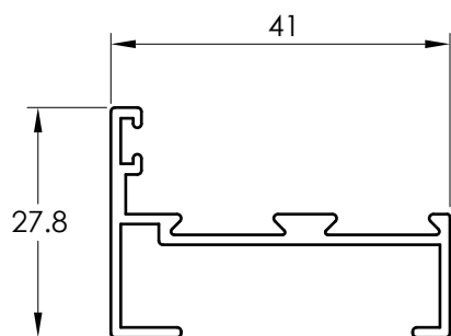
3502 MARCO
