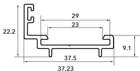
7205 TOPE SEGUNDA HOJA
