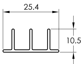
5364 DOBLE RIEL
