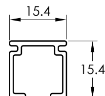
5341 RIEL CORTINA
