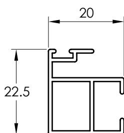
4007 TRASLAPO
