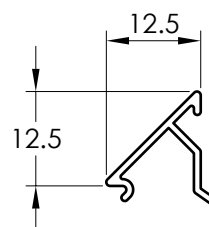
3503 JUNQUILLO 45°
