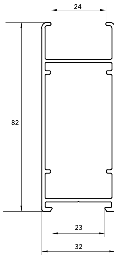
7204 BASTIDOR GRANDE TERMOPANEL
