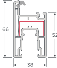
Hoja Corredera Andes 66
