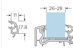
Con junquillo 17-20 Sliding Acristalamiento 26-28
