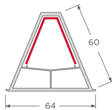
compatible con perfiles S60 Esquinero 45° S60
