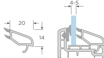
Junquillo Monolítico 4-5mm Andes
