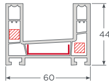
Marco Doble Riel Corredera Andes
