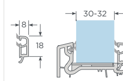
Con junquillo 20-22 Sliding Acristalamiento 30-32
