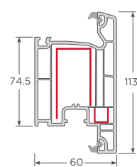
Hoja Puerta Exterior
