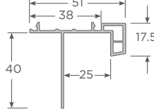
Aleta Siding Marco Fijo Andes
