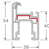
Hoja Andes 54 Blanco
