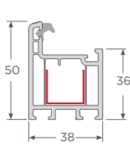
Marco Fijo Andes S38
