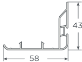
Traslapo Corredera 80 S75
