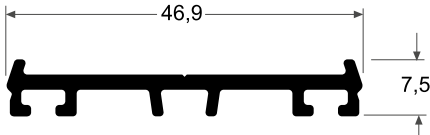
5064 Contratapa 0.374 kg/m
