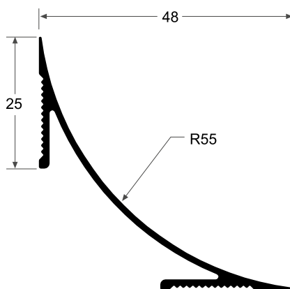
GS48 Guardapolvo Sanitario 0.362 kg/m
