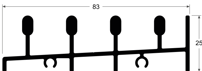
S831 Riel Inferior 4L 1.254 kg/m
