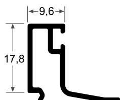
S387 Junquillo TP 0.201 kg/m
