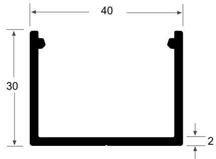
U40 Canal 40 x 30 0.541 kg/m
