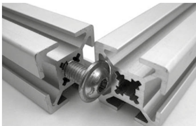
Tornillo Especial M8 x 25 mm
