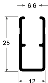
1204 Bastidor 0.220 kg/m
