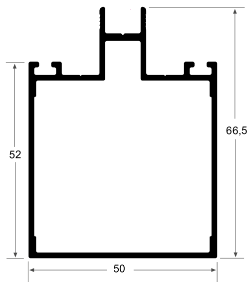
5074 Travesaño 1.032 kg/m
