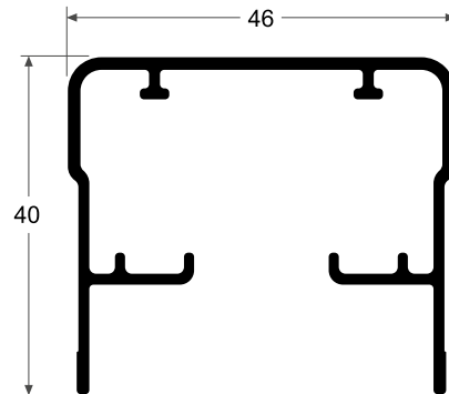
1203 Riel Superior 0.576 kg/m
