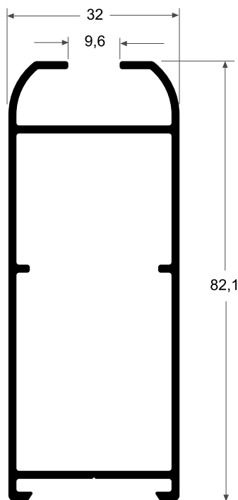
3235 Bastidor Grande 1.001 kg/m
