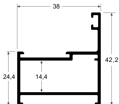
S381 Marco 0.567 kg/m
