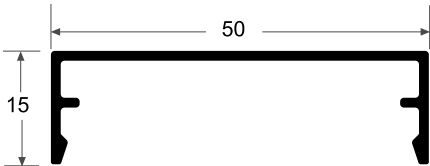
5075 Tapa 0.302 kg/m
