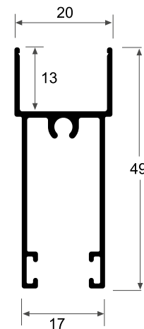
2018 Zócalo / Cabezal TP 0.419 kg/m
