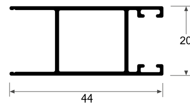
2020 Pierna Abierta TP 0.401 kg/m
