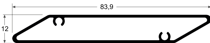
BRIRBD BRISE ROMBOIDE 84 0.609 kg/m
