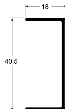
1202 Jamba 0.262 kg/m
