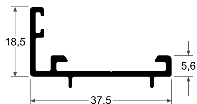
3223 Tope 2ª Hoja 0.317 kg/m
