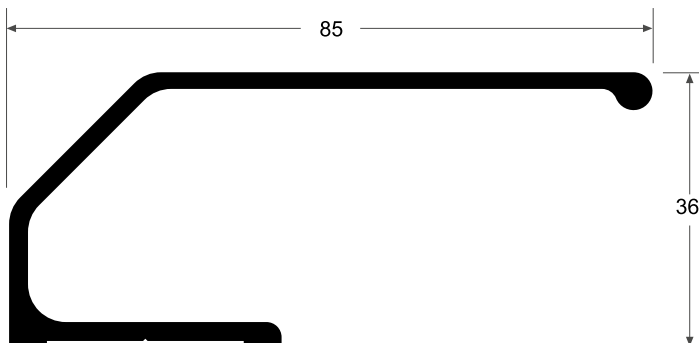
3820 Tirador 0.959 kg/m
