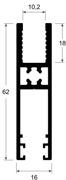
S834 Zócalo 0.907 kg/m
