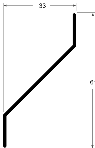
5371 Quiebravista Chico 0.300 kg/m
