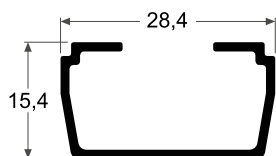
3321 Adaptador Monolítico 0.222 kg/m
