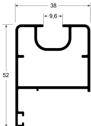
S382 Hoja 0.732 kg/m
