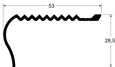
5367 Nariz de Grada 0.373 kg/m
