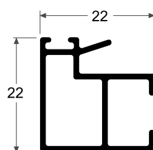
4806 Traslapo 0.269 kg/m
