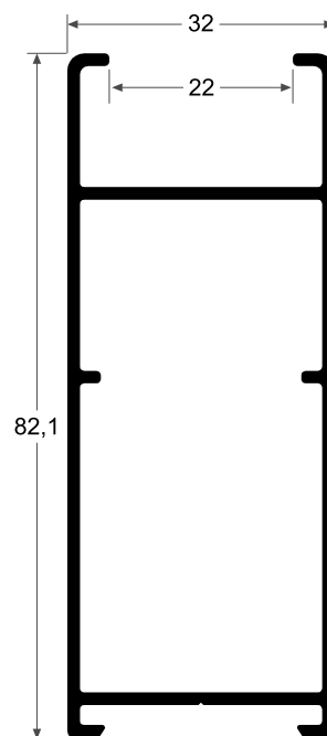
3227 Bastidor Grande TP 0.973 kg/m
