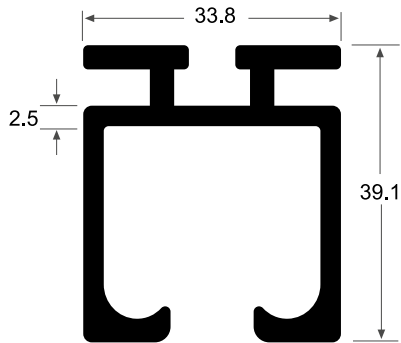
RBRI Riel Brise 1.092 kg/m
