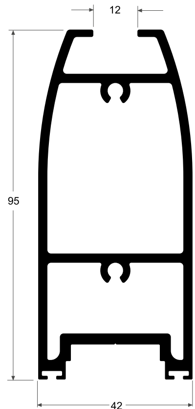
4602 Zócalo Quicio MAB 2.098 kg/m
