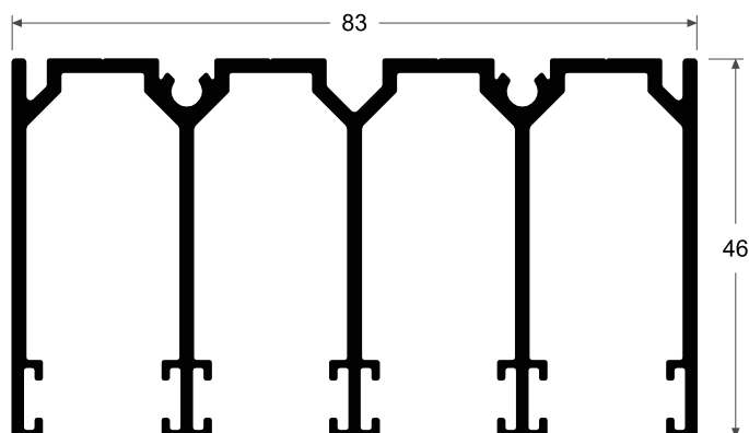
S832 Riel Superior 1.725 kg/m
