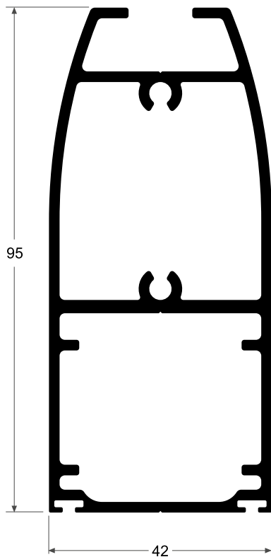
4603 Zócalo Quicio Scanavini 1.827 kg/m
