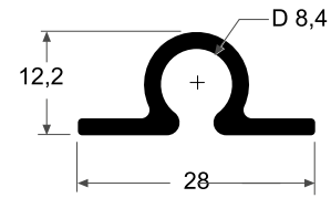
CH-215 Base Picaporte 0.268 kg/m
