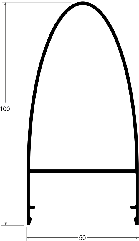
5065 Tapa Rodón 1.067 kg/m
