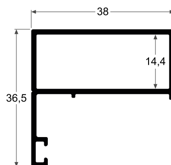
S389 Hoja Proyectante VHB 0.502 kg/m
