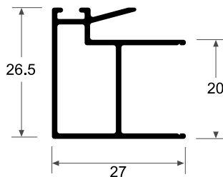
2016 Traslapo TP 0.340 kg/m
