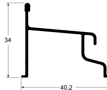
1201 Riel Inferior 0.356 kg/m
