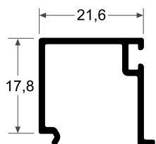
S383 Junquillo 0.208 kg/m
