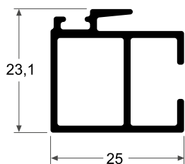
5006 Traslapo 0.330 kg/m
