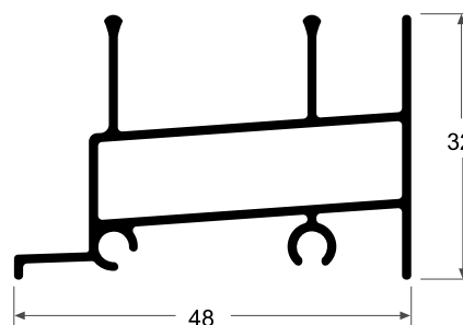
4812 Riel Cámara 0.544 kg/m
