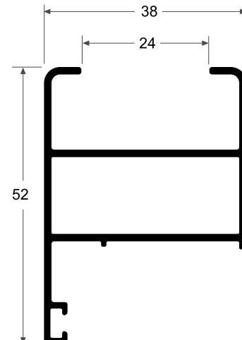
S386 Hoja TP 0.655 kg/m
