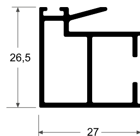
2019 Traslapo 0.403 kg/m
