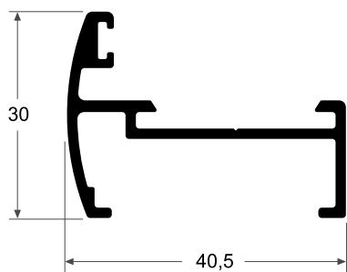
3222 Marco 0.468 kg/m
