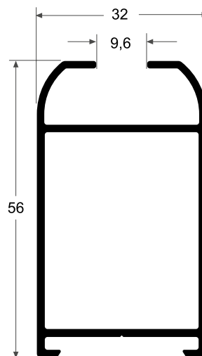
3221 Bastidor Chico 0.746 kg/m
