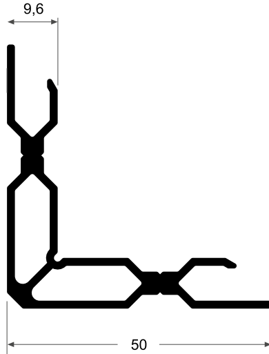
4220 Escuadra Tubular 0.813 kg/m
