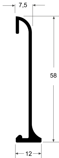
5366 Guardapolvo 0.353 kg/m
