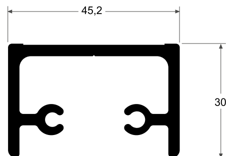
5059 Soporte 1.062 kg/m
