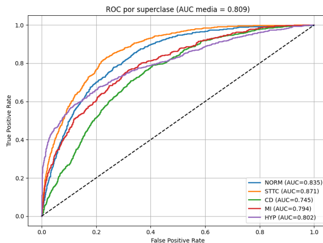
Figura 6.8: Conjunto de ROCs de random forest de la configuración 1 (Características)
