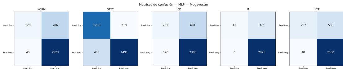
Figura 6.9: Matrices de confusión de red neuronal de la configuración 1 (Megavector)
