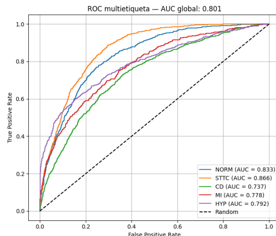
Figura 6.6: Conjunto de ROCs de random forest de la configuración 1 (Megavector)
