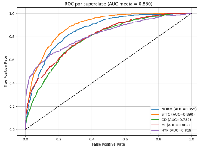
Figura 6.12: Conjunto de ROCs de red neuronal de la configuración 1 (Características)
