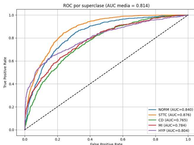
Figura 6.10: Conjunto de ROCs de red neuronal de la configuración 1 (Megavector)
