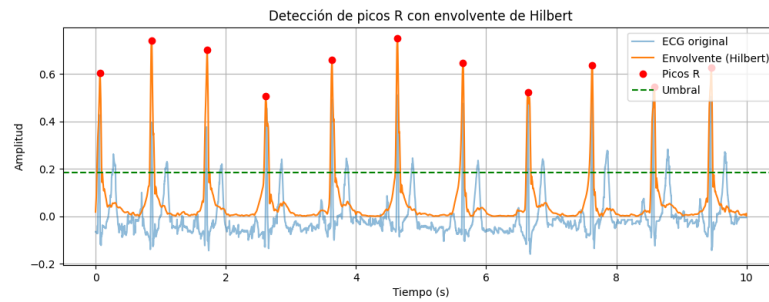
Figura 5.13: Picos R detectados en la envolvente.
