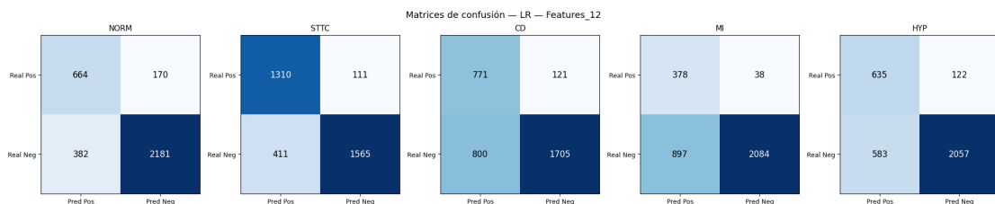
Figura 6.13: Matrices de confusión de regresión logística de la configuración 2
