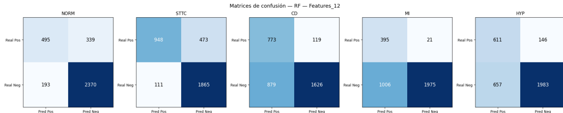
Figura 6.15: Matrices de confusión de random forest de la configuración 2
