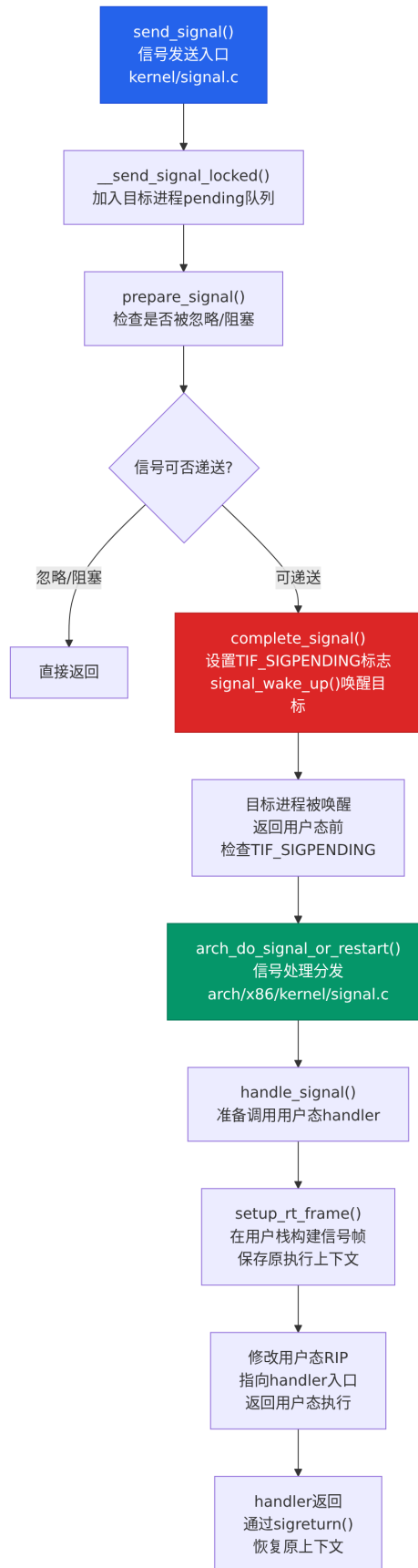
图 7: Linux 信号发送与处理流程
