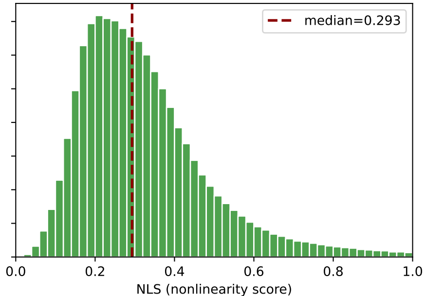
Wikitext-103 GPT-2-small MLP (layer 0)
