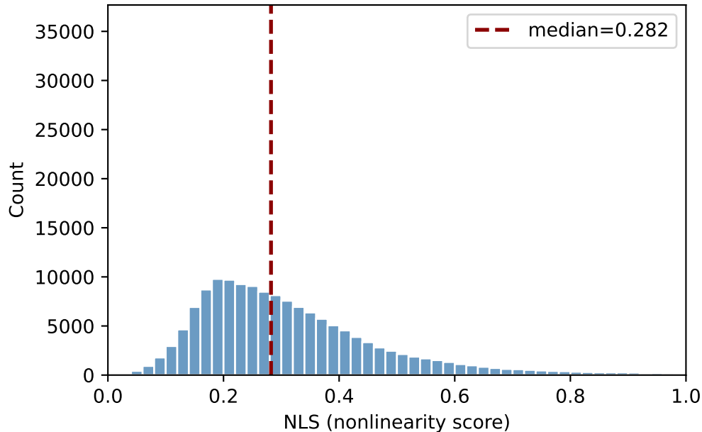
GuppyLM MLP (layer 0)
