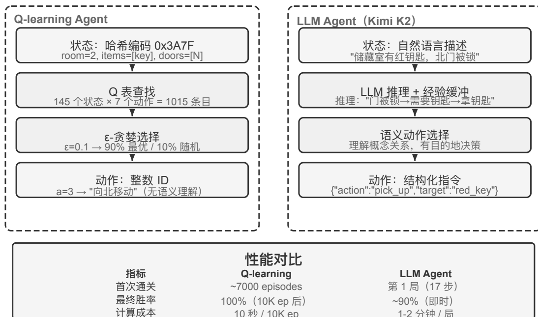
图 7-7 Q-learning 与 LLM Agent 在寻宝游戏中的架构对比
