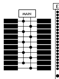
TLM2012CCURP
