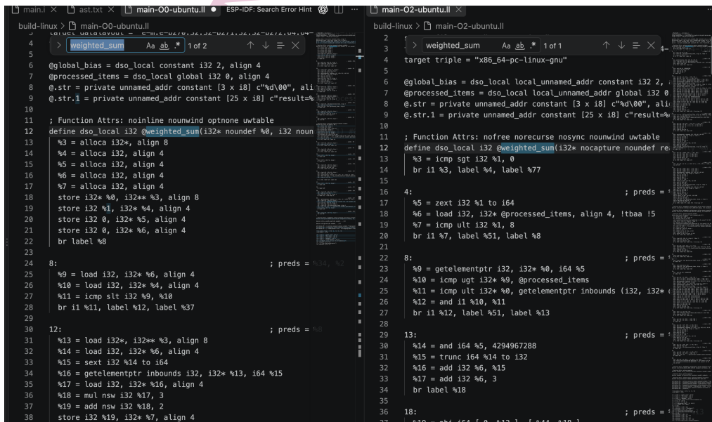
图 39 同一函数在 -O0 与 -O2 下的 LLVM IR 对照
