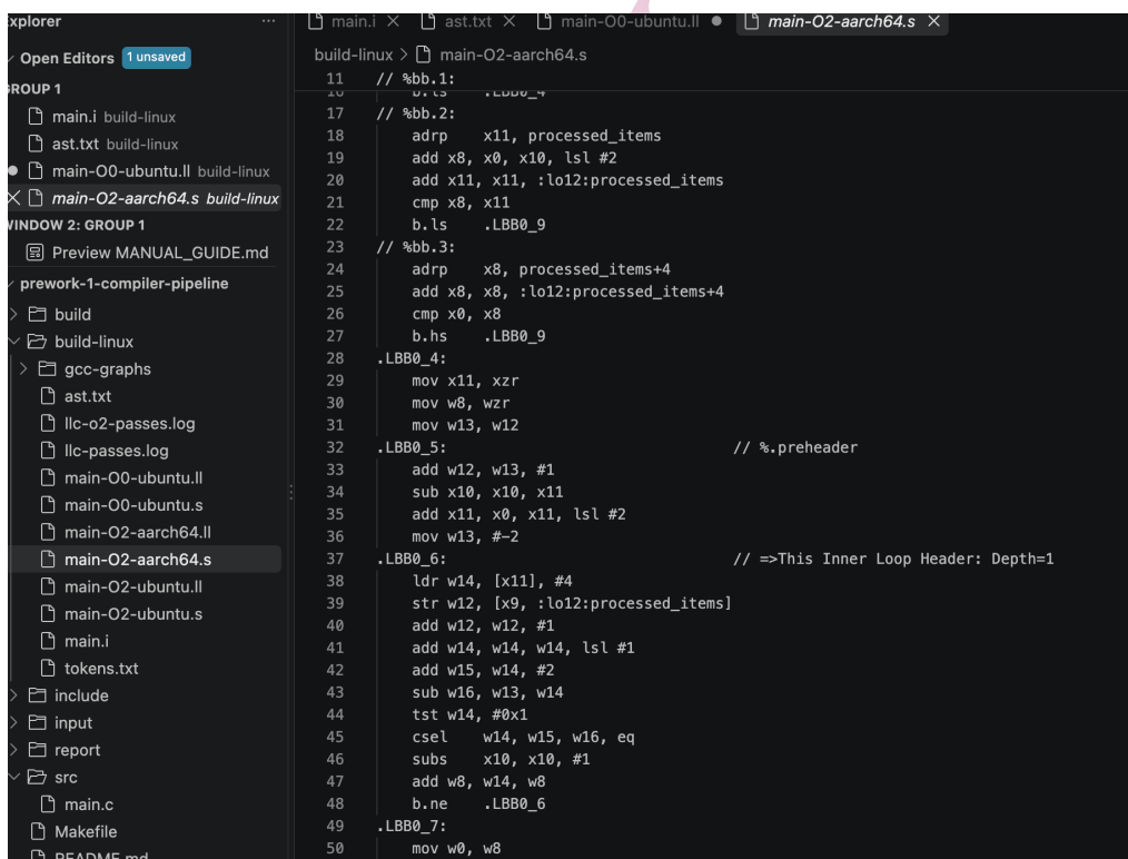
图 40 LLVM 后端生成的 AArch64 汇编
