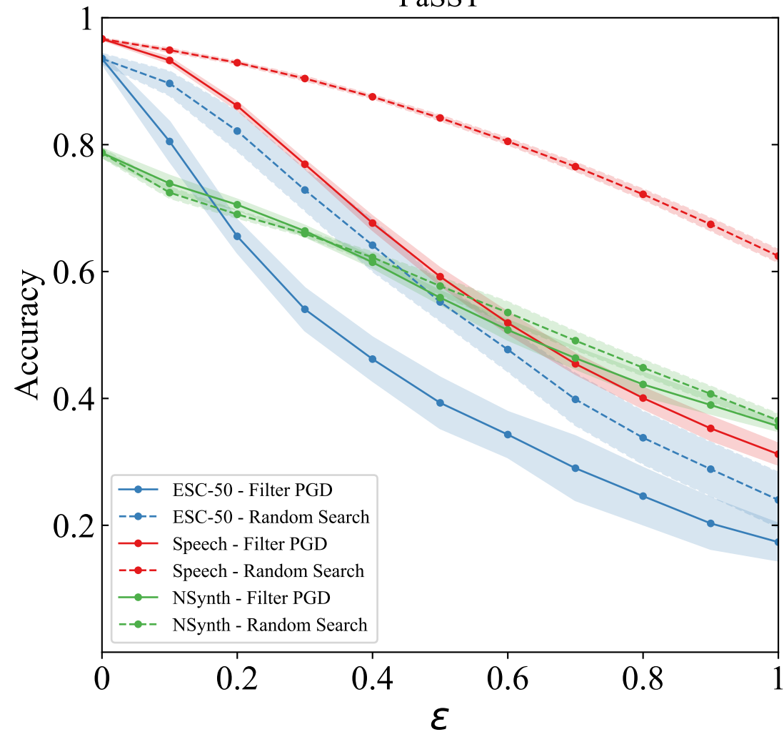
PaSST
