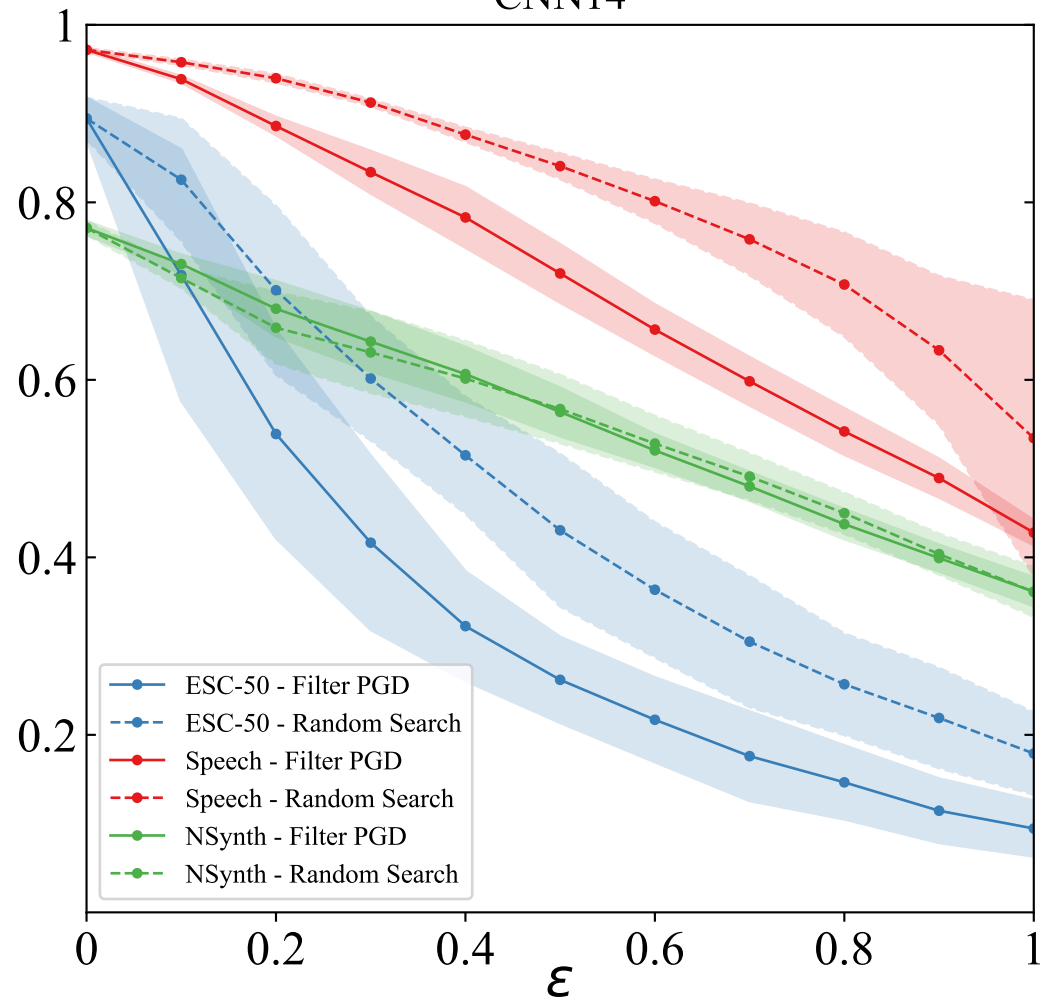
CNN14
