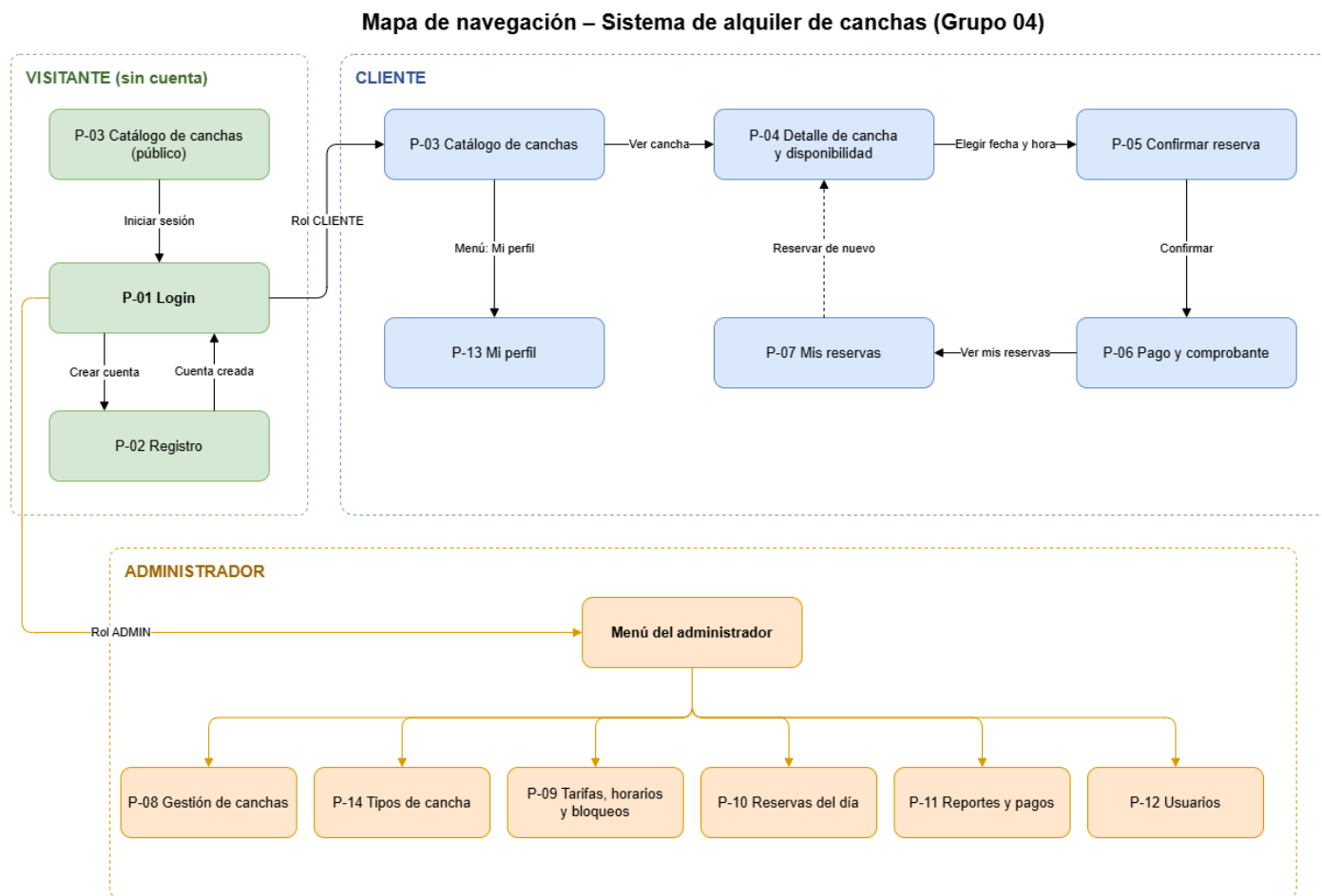
Fig. 1. Mapa de navegación del sistema Golazo por tipo de usuario.
