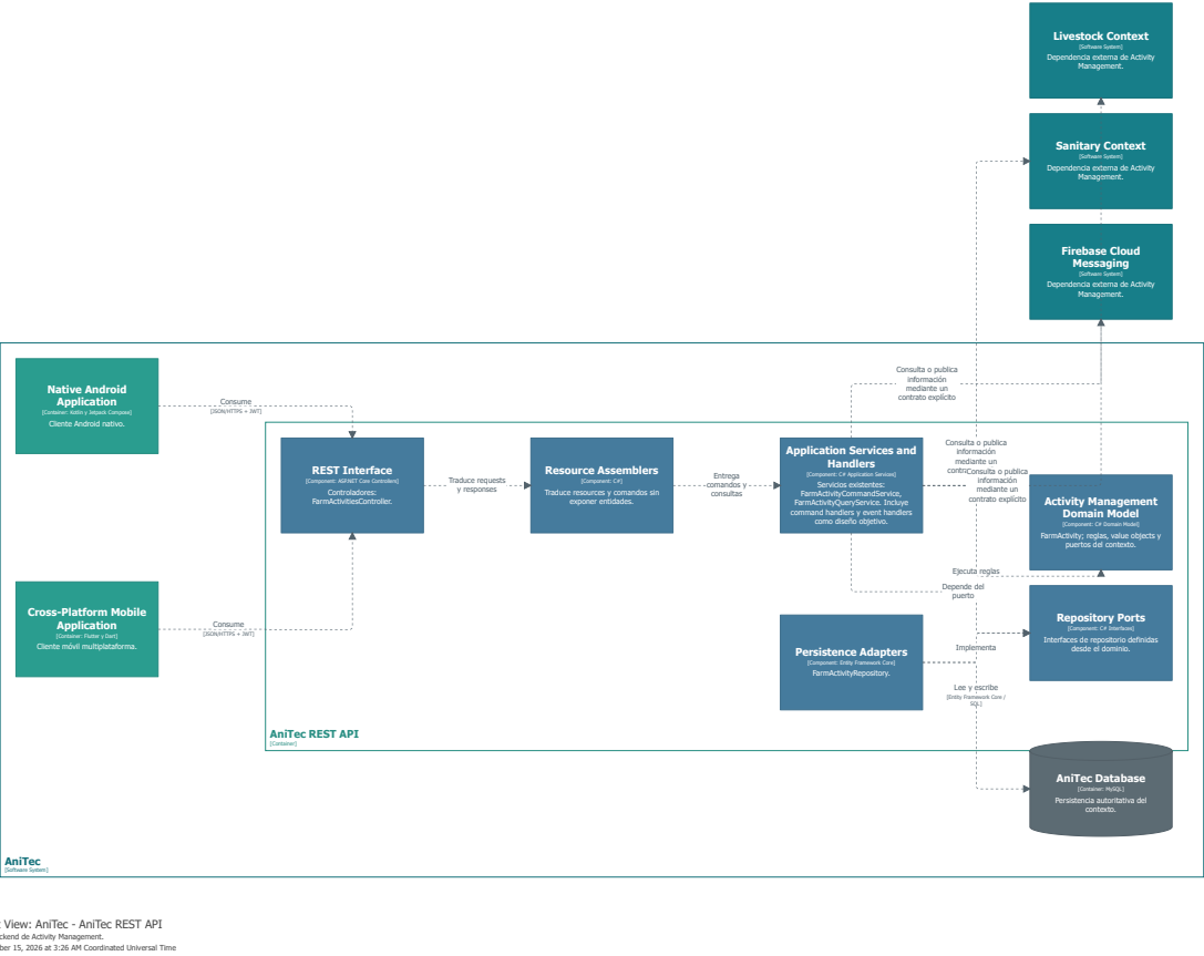
Figura 2.6.6.1. Componentes de la API para Activity Management. Fuente: elaboración propia con Structurizr DSL.
