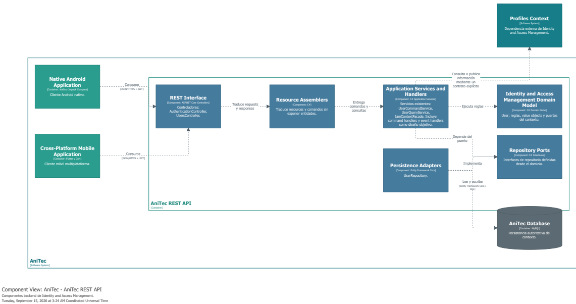
Figura 2.6.1.1. Componentes de la API para Identity and Access Management. Fuente: elaboración propia con Structurizr DSL.
