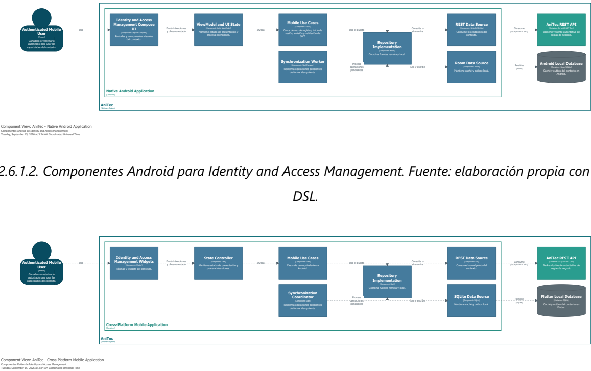
Figura 2.6.1.3. Componentes Flutter para Identity and Access Management. Fuente: elaboración propia con Structurizr DSL.
