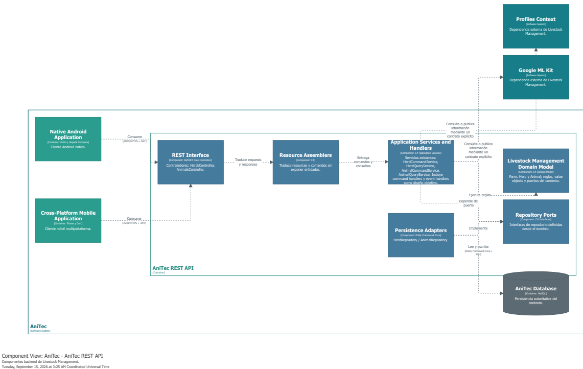
Figura 2.6.3.1. Componentes de la API para Livestock Management. Fuente: elaboración propia con Structurizr DSL.
