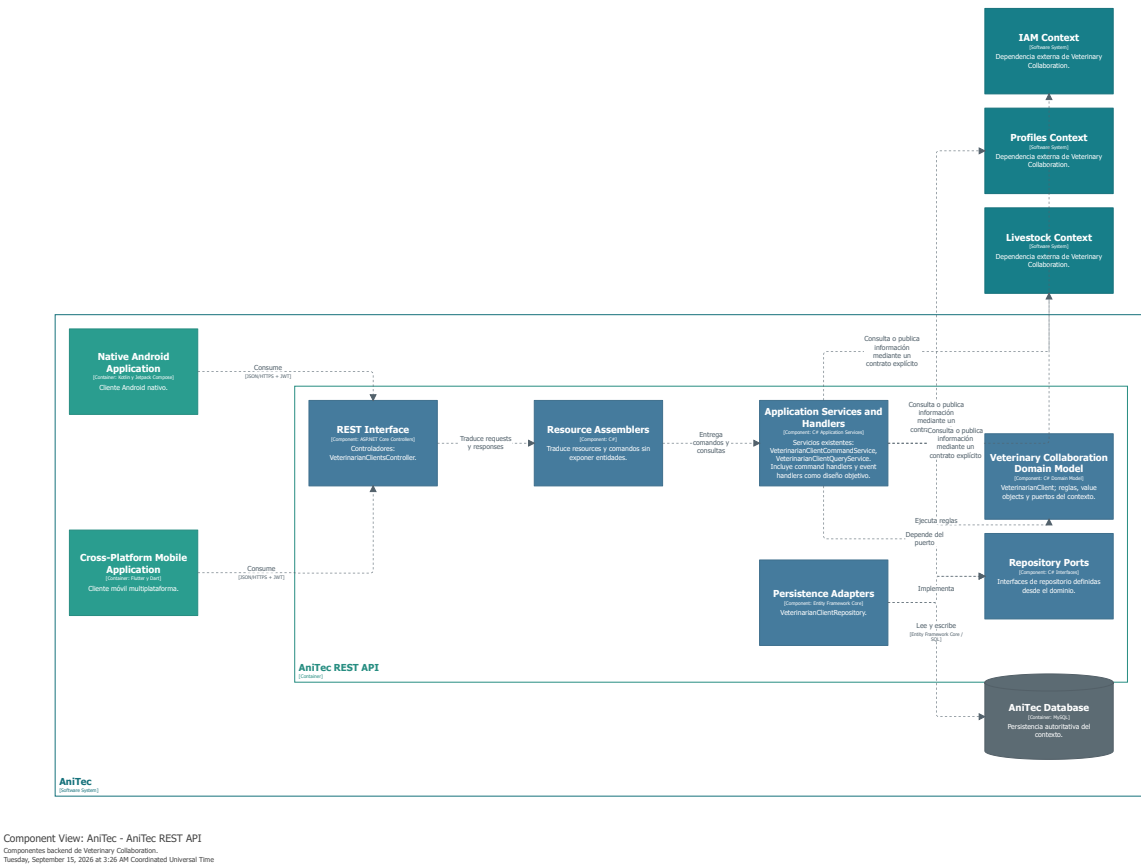
Figura 2.6.5.1. Componentes de la API para Veterinary Collaboration. Fuente: elaboración propia con Structurizr DSL.
