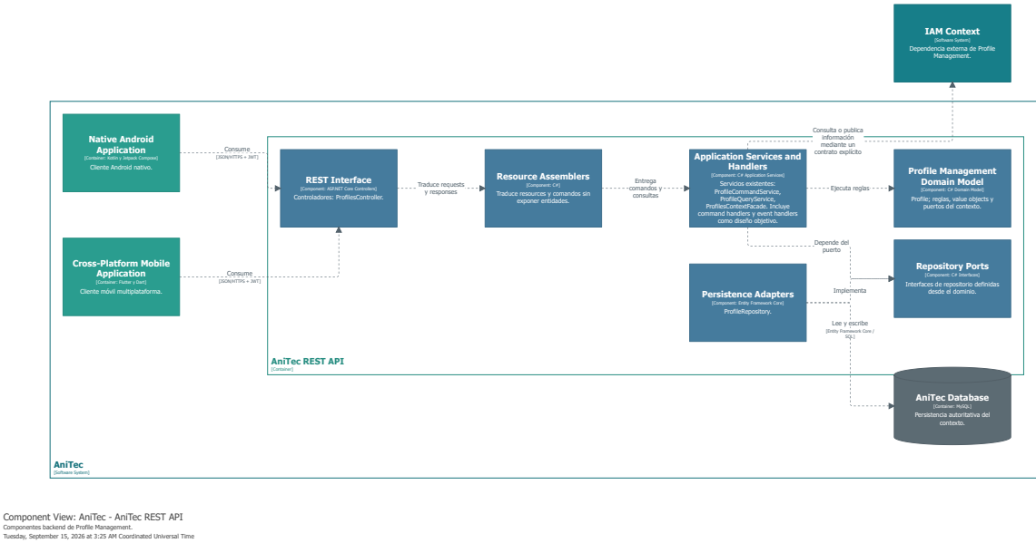
Figura 2.6.2.1. Componentes de la API para Profile Management. Fuente: elaboración propia con Structurizr DSL.
