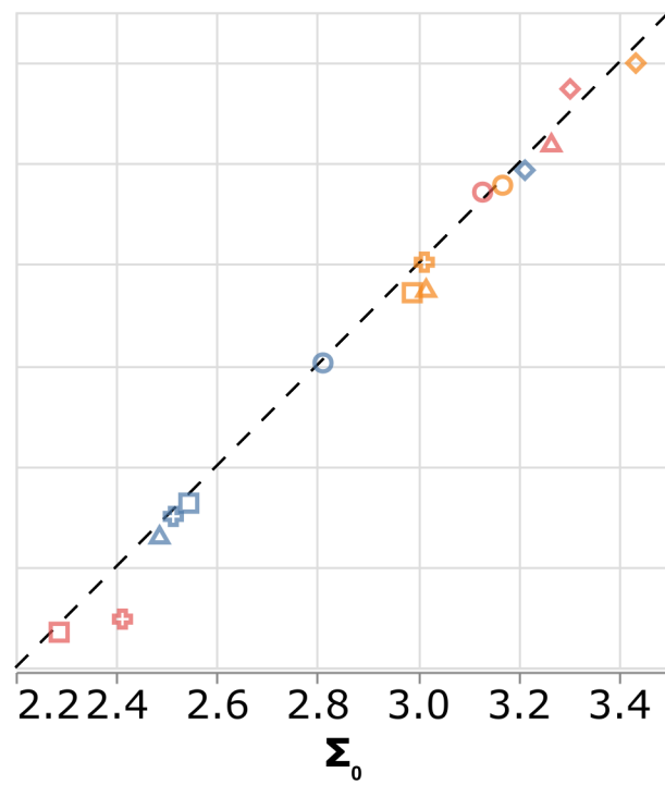
Monte Carlo (N = 100)
