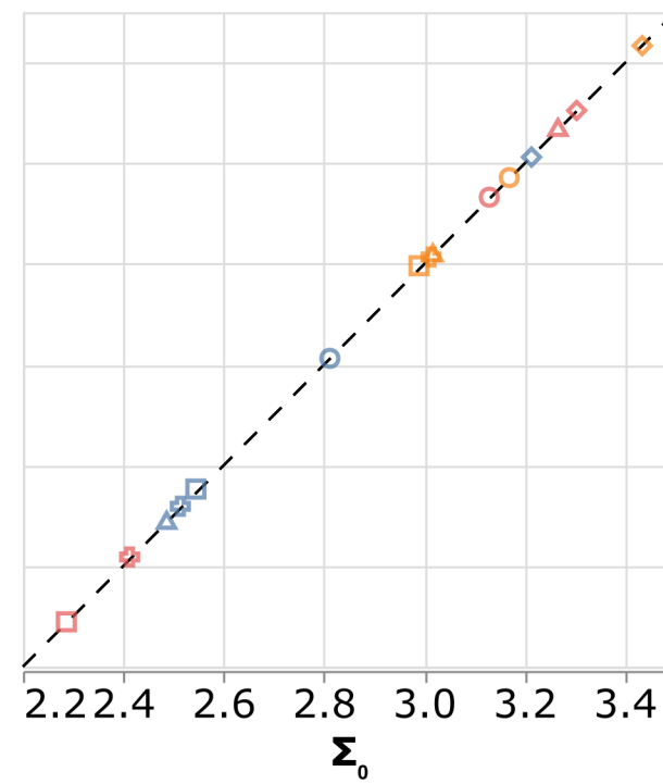
Monte Carlo (N = 10000)
