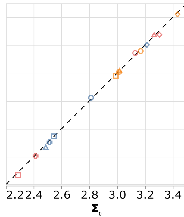
Monte Carlo (N = 1000)
