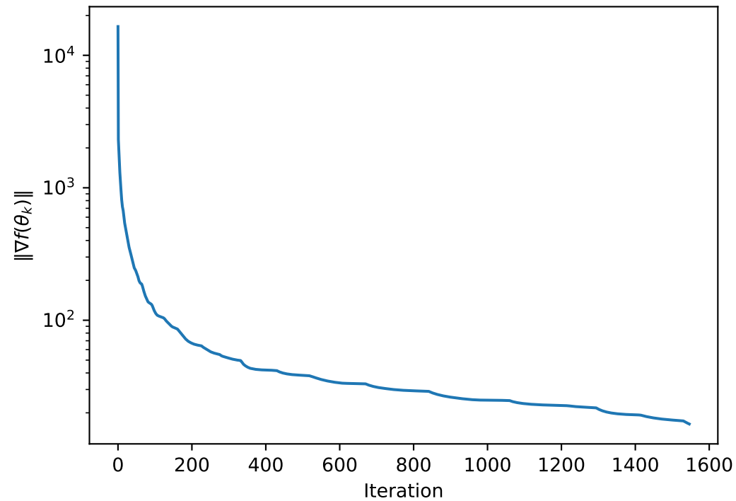
Gradient norm
