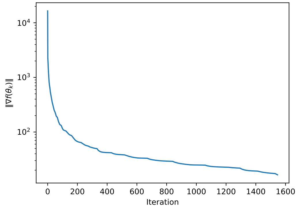
Gradient norm
