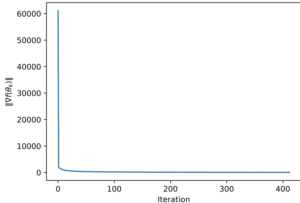
Gradient norm
