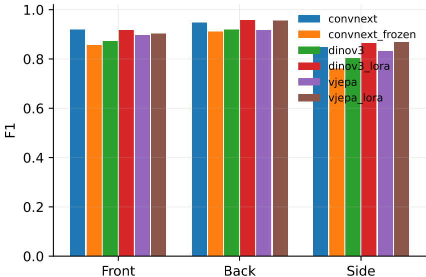
MTSD attributes - view-angle per-class F1
