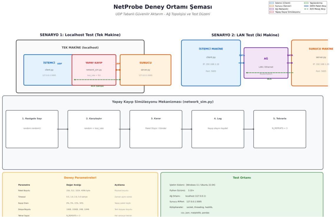
Şekil 11: Deney Ortamı Şeması
