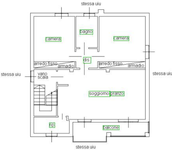
Piano Primo H=3.00m
