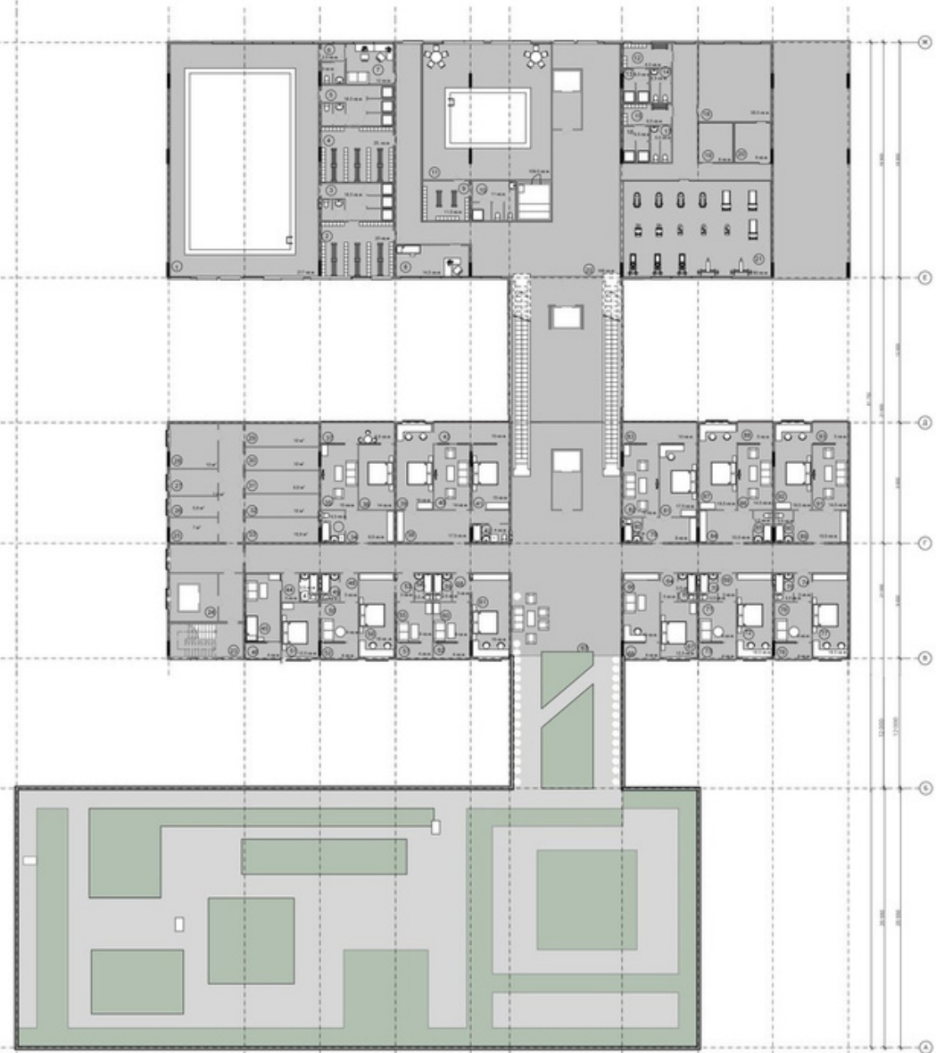
План третьего поверху М 1:200 Second floor plan 1:200
