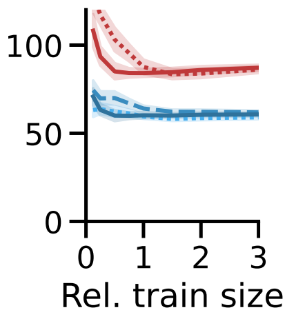
xz
