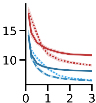
H2
