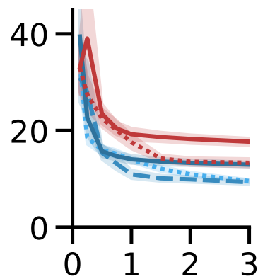
batik
