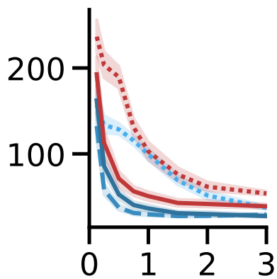
VP9
