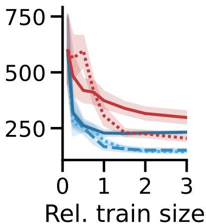
z3
