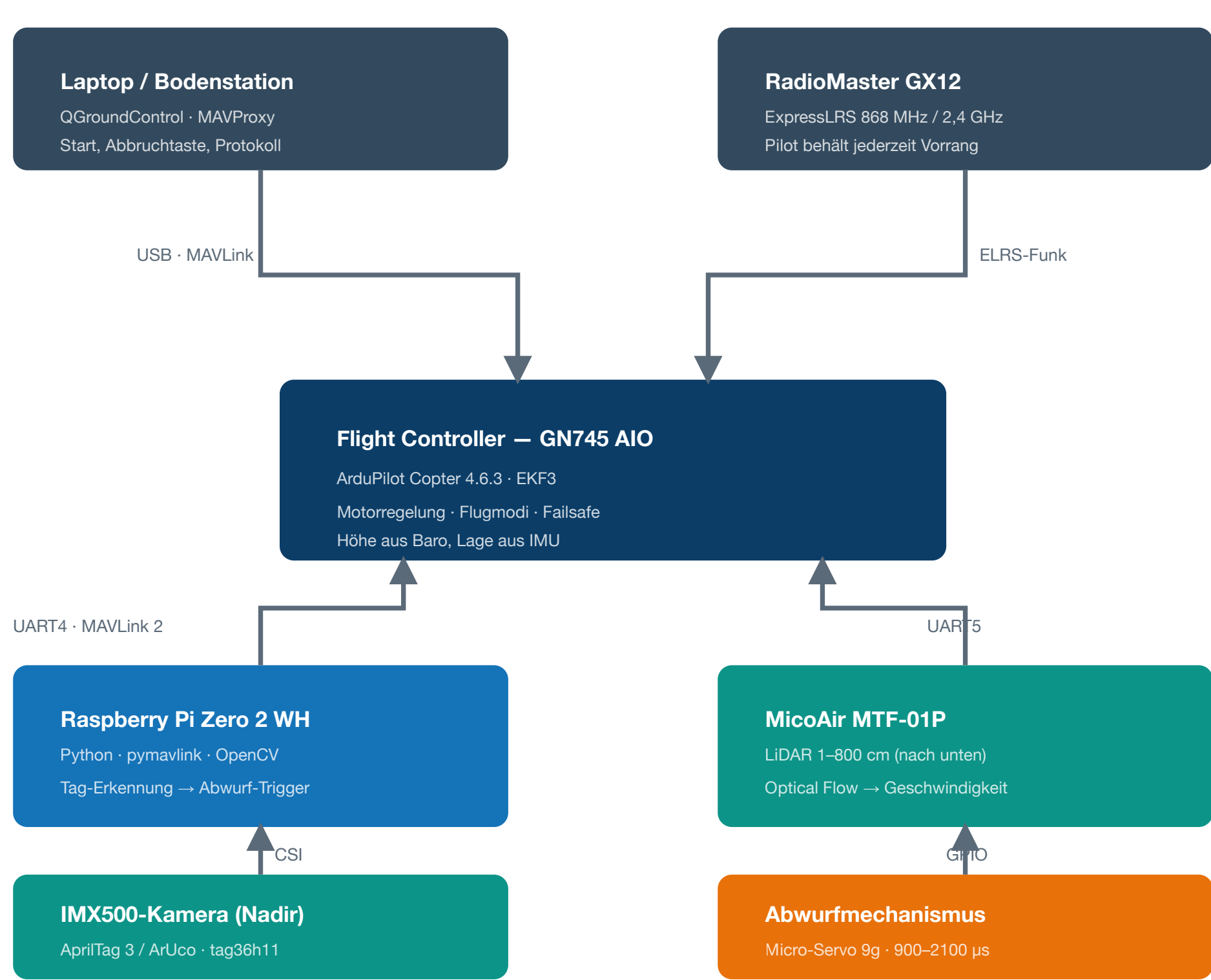
Abb. 2: Signalfluss zwischen Bodenstation, Fernsteuerung, Autopilot, Companion-Computer, Sensorik und Abwurf.
