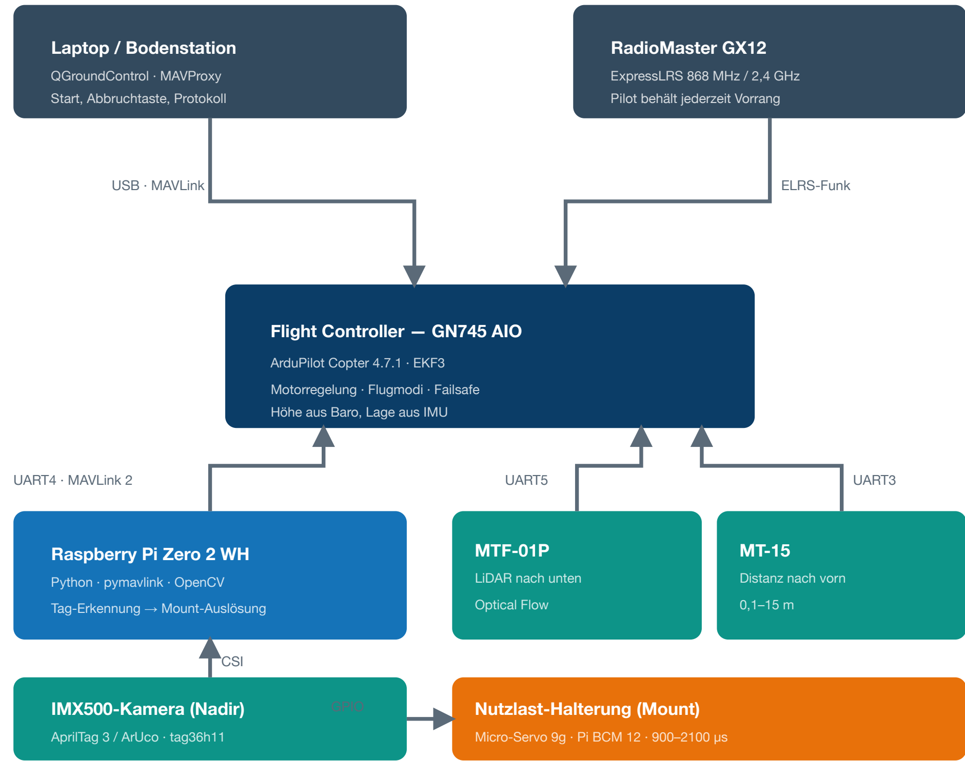
Abb. 2: Signalfloss zwischen Bodenstation, Autopilot, Companion-Computer und Sensorik.
