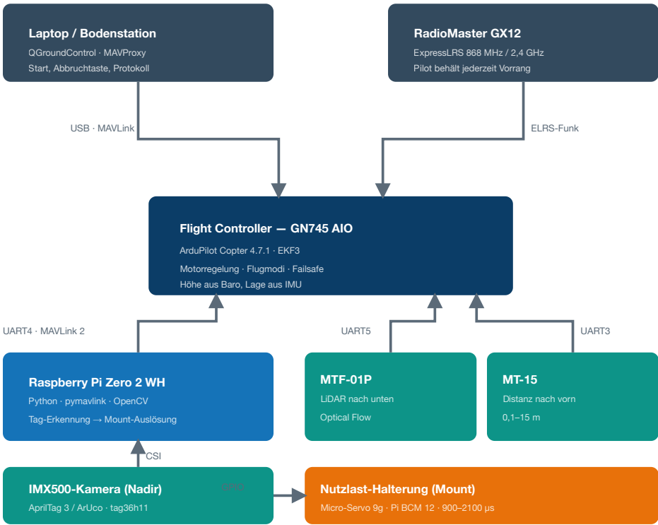
Abb. 2: Signalfloss zwischen Bodenstation, Autopilot, Companion-Computer und Sensorik.
