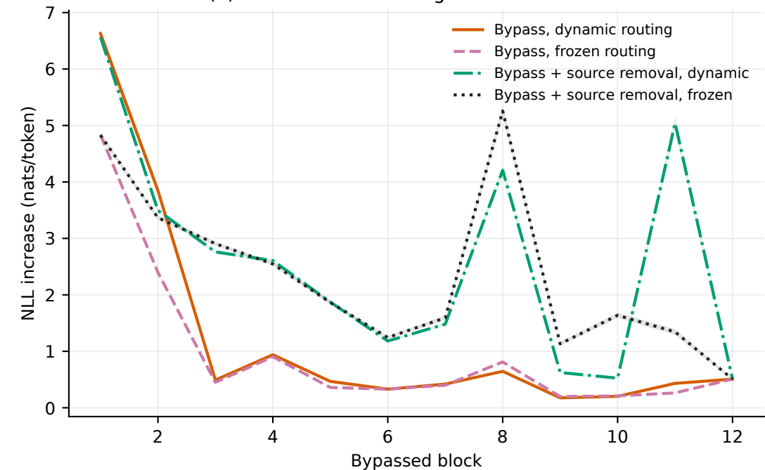
(d) DAG: effect of routing and source access
