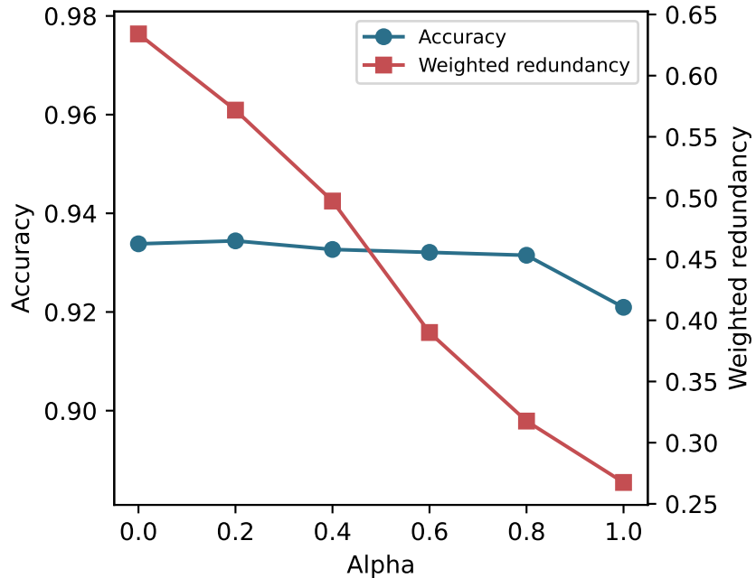
WDBC
