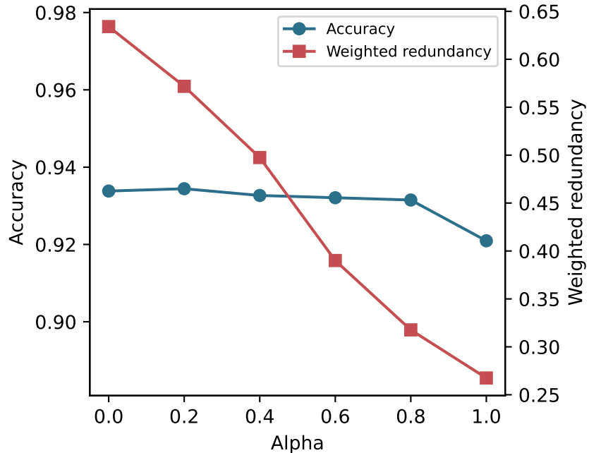
WDBC
