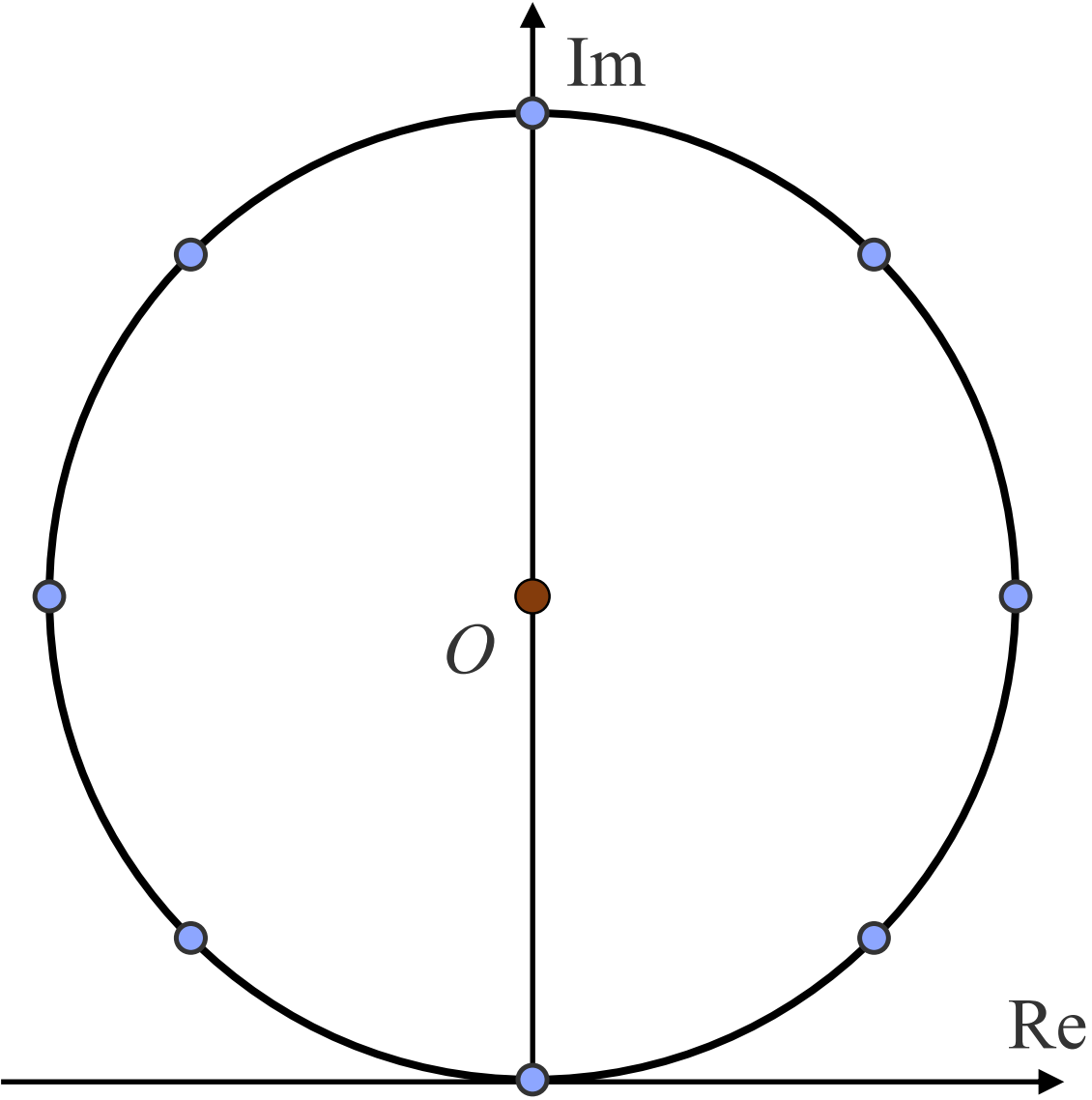
(a) 均匀离散相移
