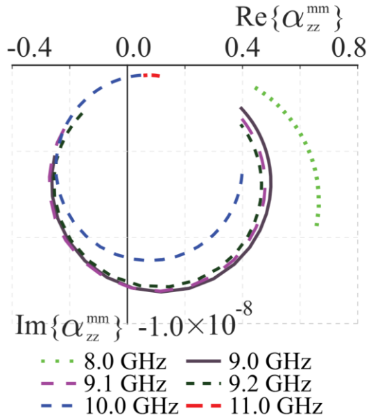
(b) 不同频率下的极化率轨迹
