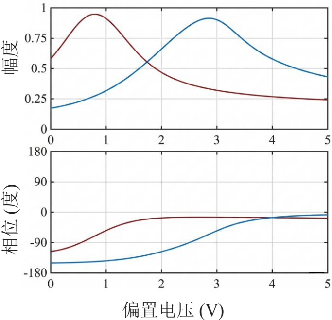
(a) 随偏置电压变化的幅度与相位响应
