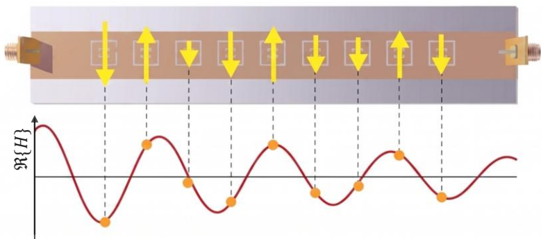
(c) 伴随波导损耗的信号传播与辐射过程
