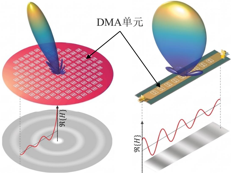
(a) 二维DMA阵列示意图
