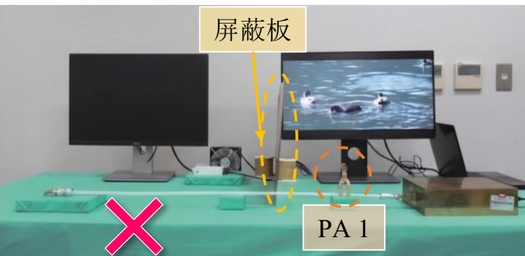
(c) 安装屏蔽板阻挡
