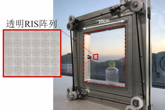
(c) 玻璃基板RIS原型
