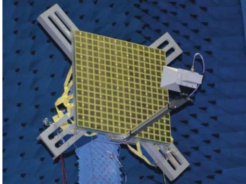
(b) 清华大学 2-bit RIS原型
