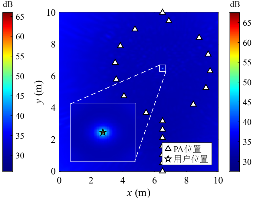
(b) 优化后圆形阵列的MUSIC空间谱
