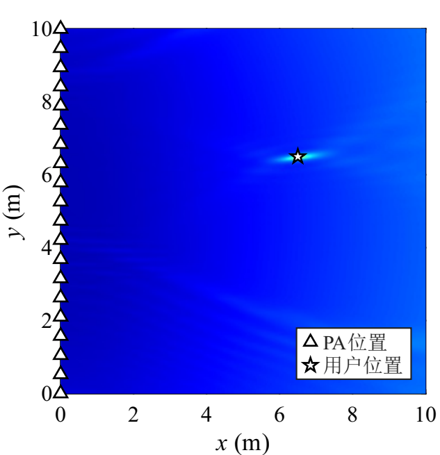
(a) 初始固定阵列的MUSIC空间谱
