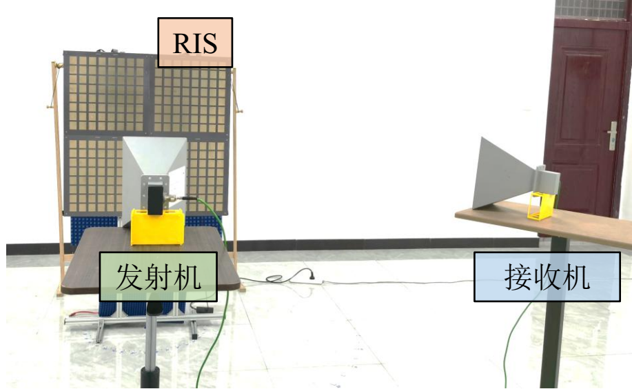
(b) 实际测试环境照片
