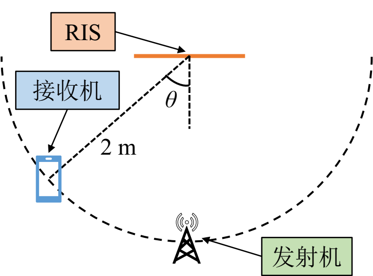
(a) RIS与收发天线位置示意图
