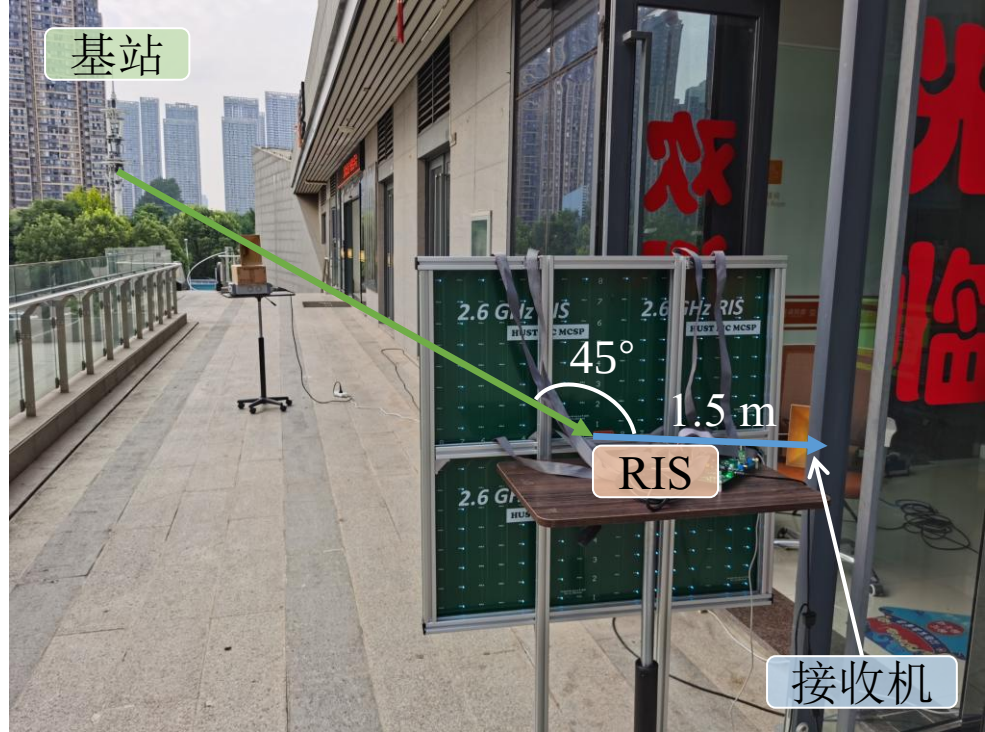
(b) RIS 面板与接收终端部署照片
