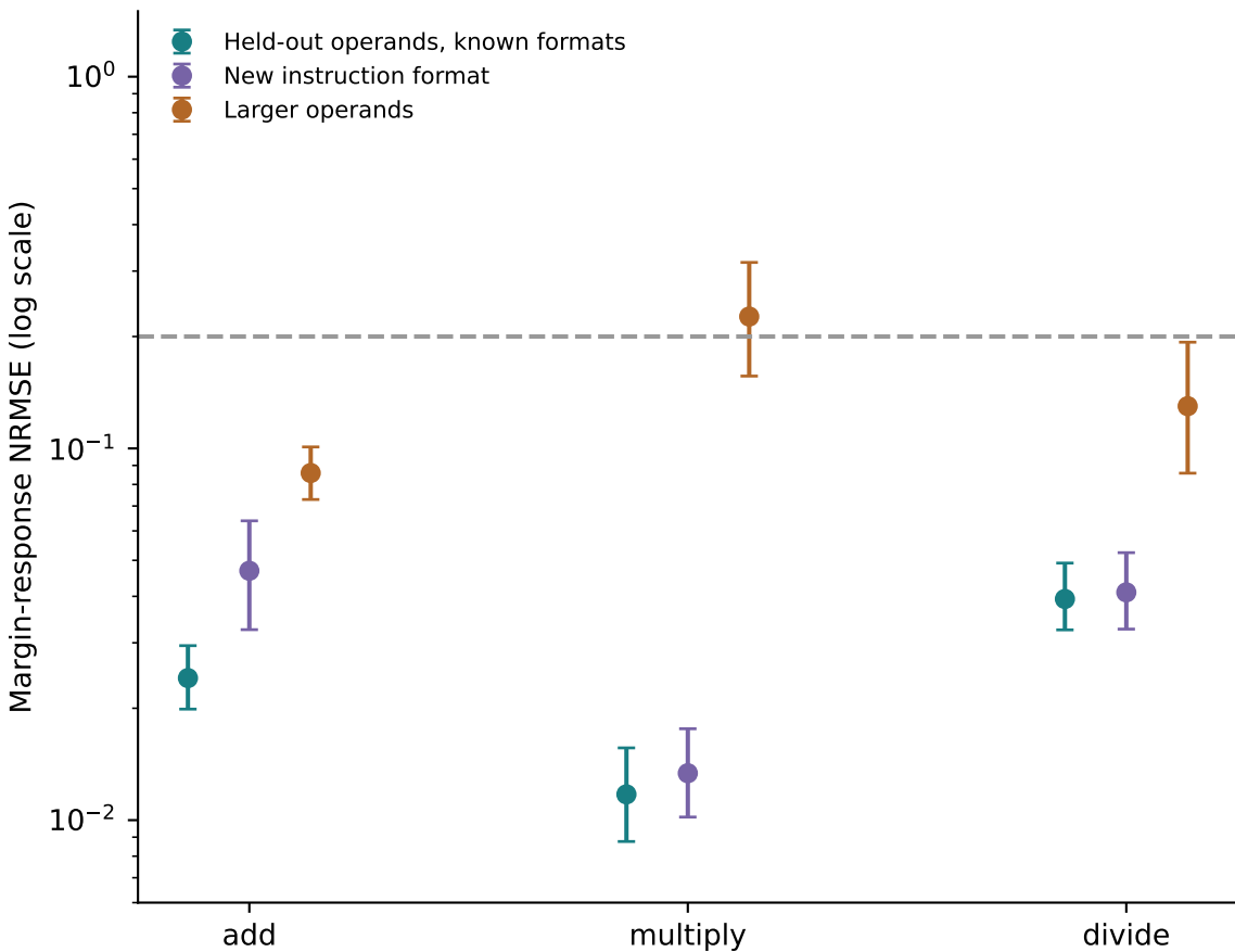
Qwen3-1.7B
