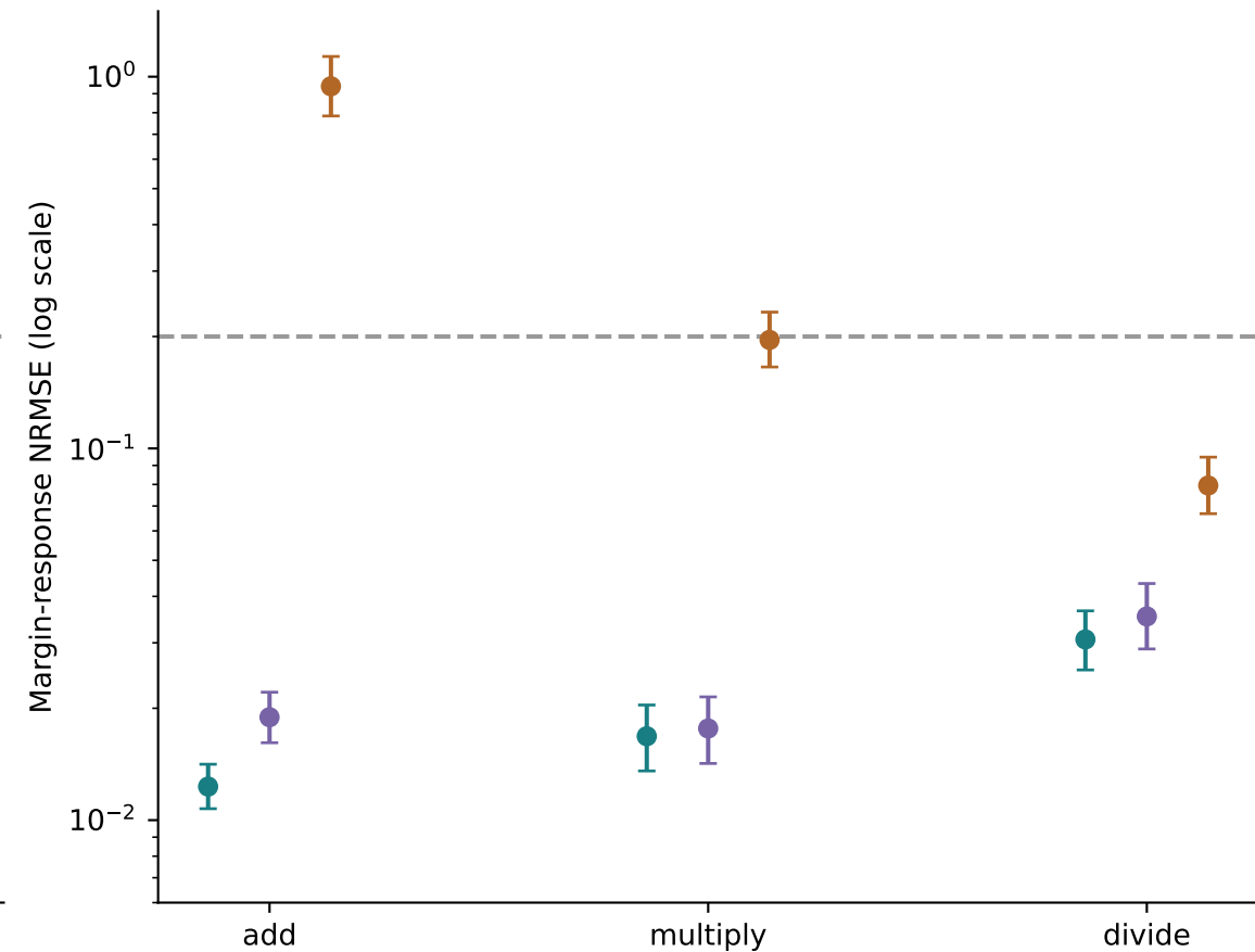
Qwen3-0.6B
