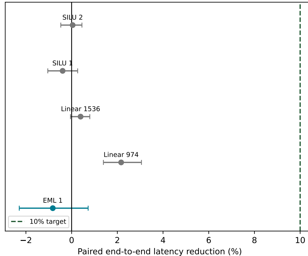
Batch 8 / prefill 512 / decode 32
