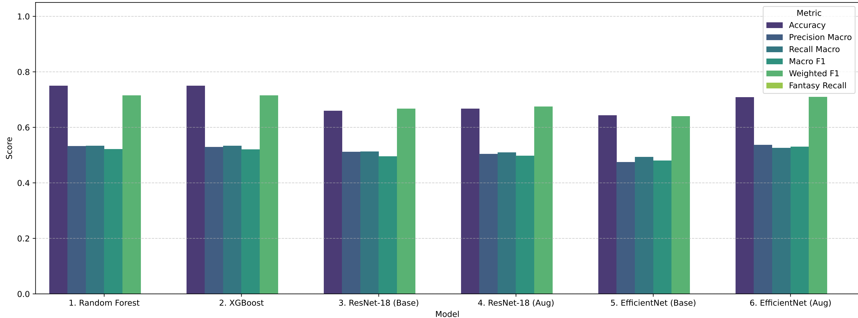
Benchmark Tipográfico - Comparação dos Modelos
