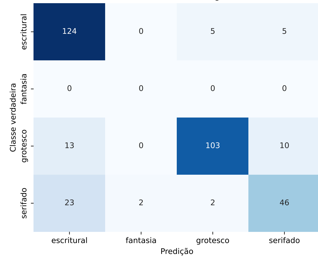
6. EfficientNet (Aug)
