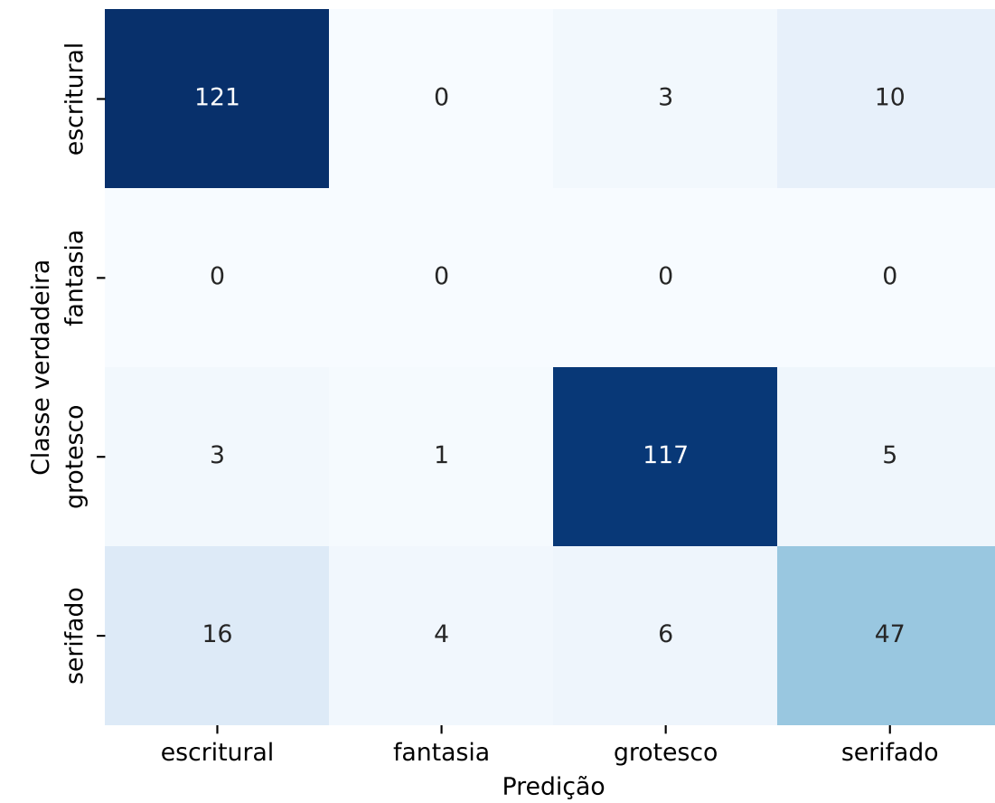
6. EfficientNet (Aug)
