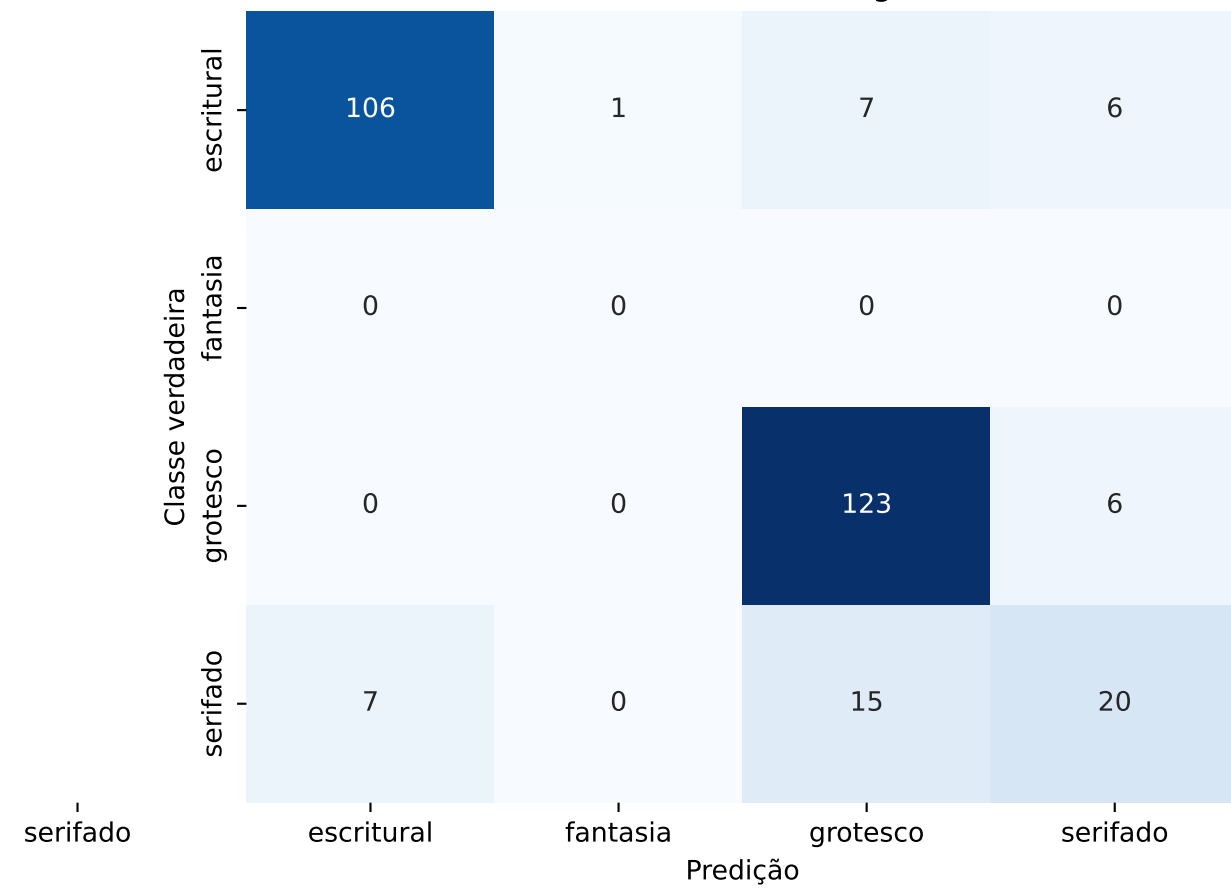
6. EfficientNet (Aug)
