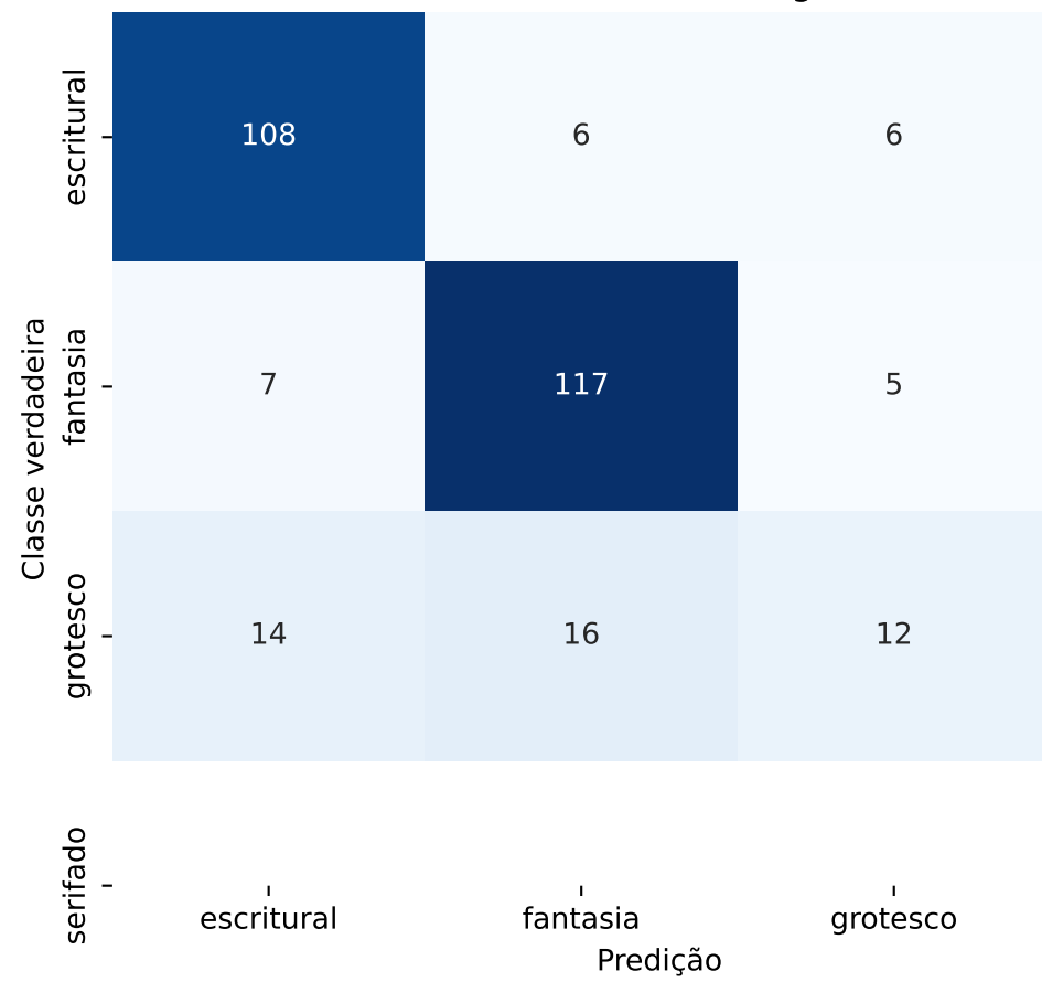
4. ResNet-18 (Aug)
