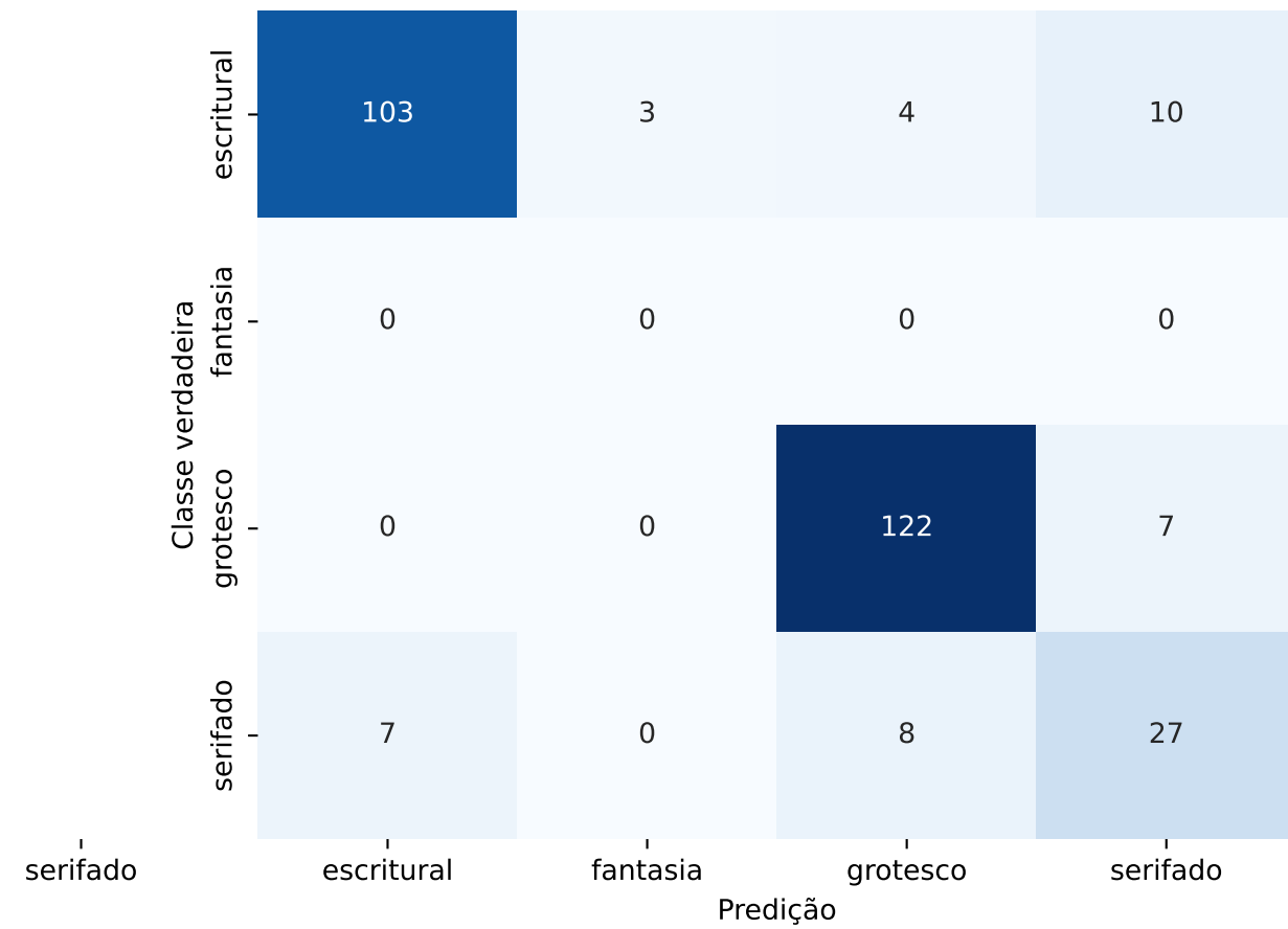
6. EfficientNet (Aug)
