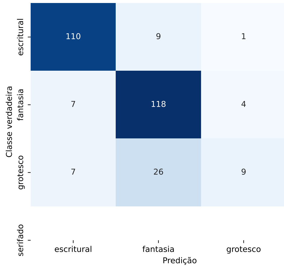
4. ResNet-18 (Aug)
