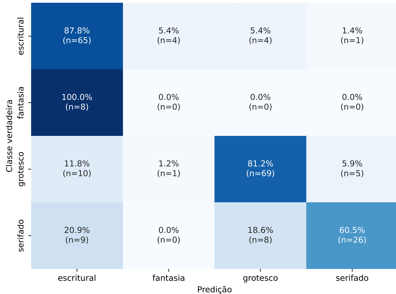
ResNet-18 (Final) — conjunto de teste
