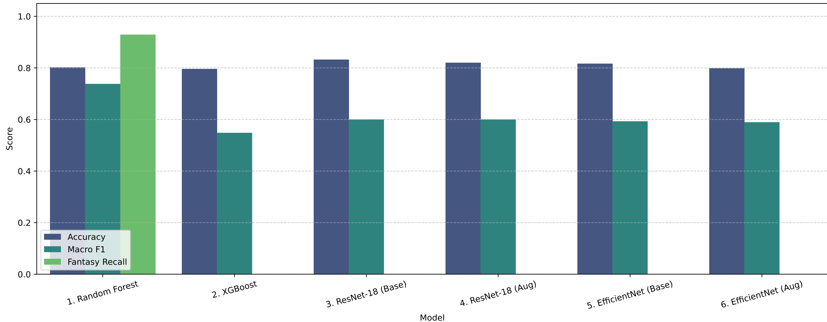
Benchmark Tipográfico: Desempenho dos 6 Modelos no Test Set
